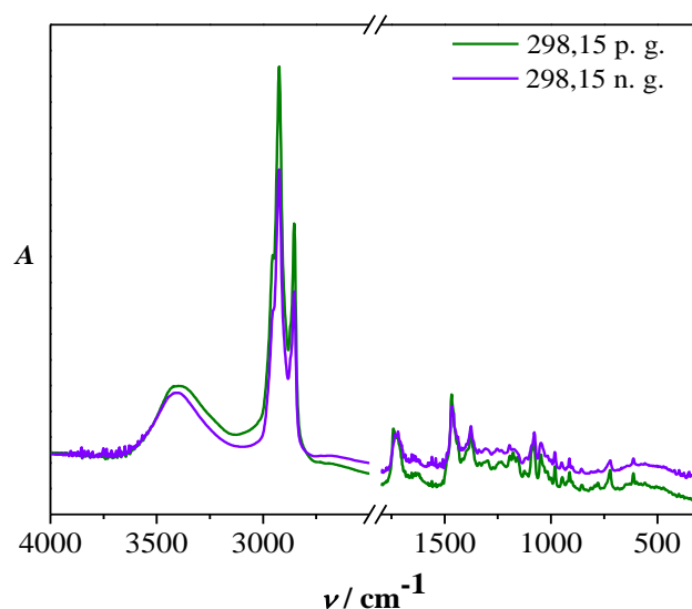
Slika 84. IR spektar TDMA–Ch snimljen prije (p.g.) i nakon (n.g.) termičkog tretmana. 285
