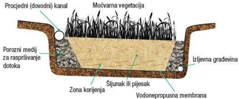
Slika 2. Biljni uređaj s horizontalnim tokom (Malus i Vouk 2012)
