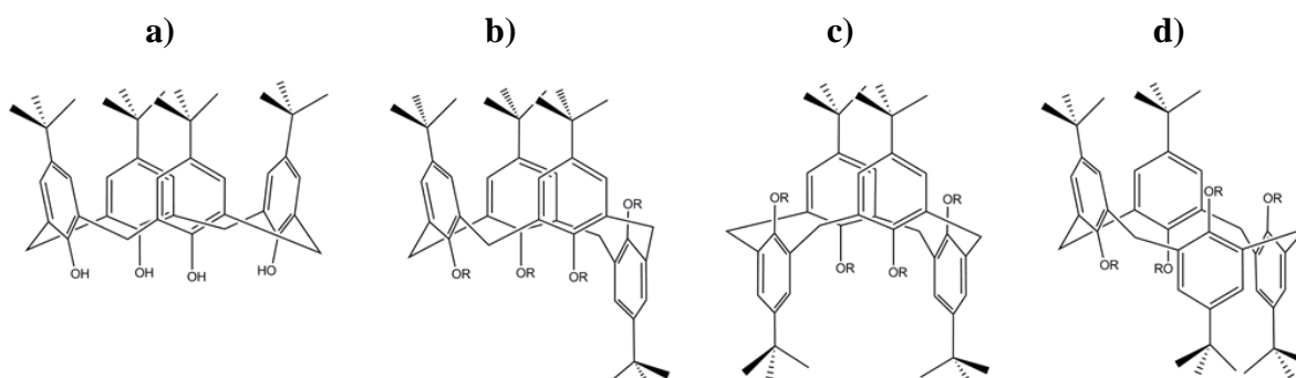
Slika 8. Konformacije kaliks[4]arena: a) stožac , b) djelomičan stožac , c) 1,3-naizmjeničan stožac , d) 1,2-naizmjeničan stožac .
