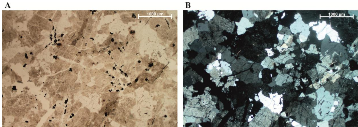
Slika 4.2: (A) Mikroskopski izgled granita: zrnata struktura s hipidiomorfim do alotriomorfim zrnima feldspata i kvarca. Granice među zrnima jasno su izražene zbog kaolinitizacije feldspata, dok je kvarc netrošan. N-. (B) N+.
