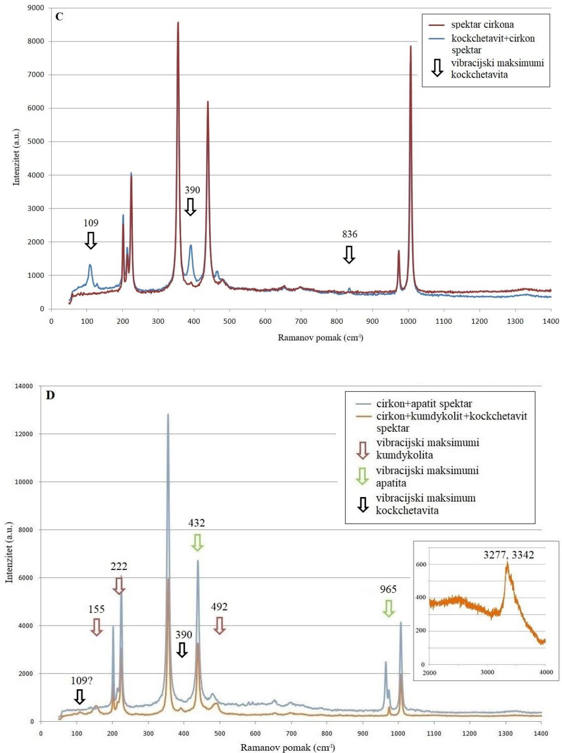
Slika 4.11: (A) Raman spektar hematita u zrnu cirkona. Vibracijski maksimum hematita na 223 cm -1 moguće se preklapa s maksimumom cirkona. (B) Raman spektar apatita u zrnu cirkona, u isječku maksimum apatita na većim vrijednostima Ramanovog pomaka. (C) Raman spektar kockchetavita u zrnu cirkona. (D) Raman spektar apatita, kumdykolita i kockchetavita u zrnu cirkona. Vibracijski maksimum apatita na 432 cm -1 preklapa se s maksimumom cirkona. U isječku maksimum apatita na većim vrijednostima Ramanovog pomaka.
