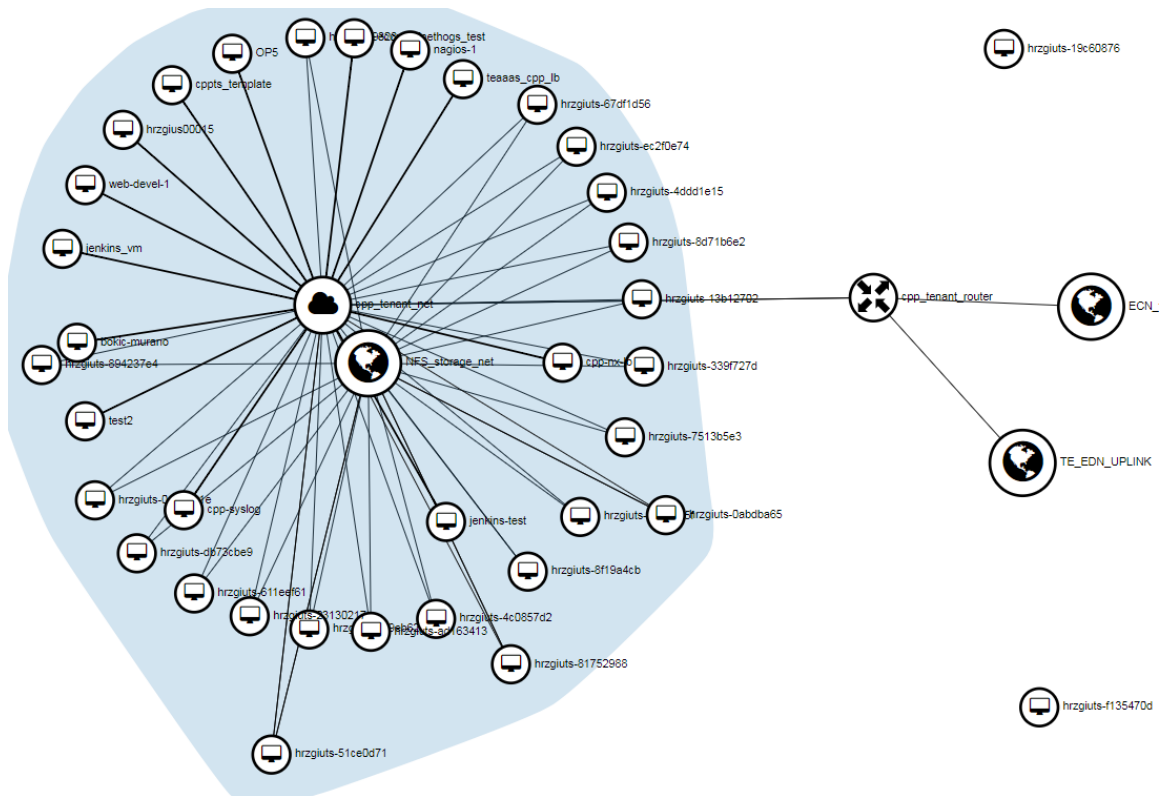
Slika 4.22: Struktura mreže u OpenStack projektu CPP_tenant
