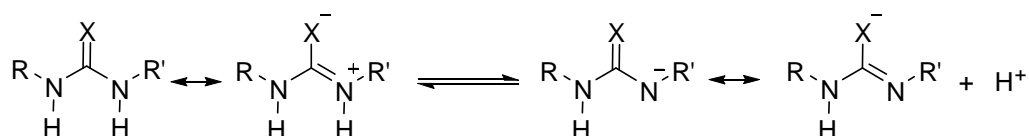
Slika 88. Shematski prikaz disocijacije ureidnih ( X = O ) i (tio)ureidnih ( X = S ) derivata. 101
