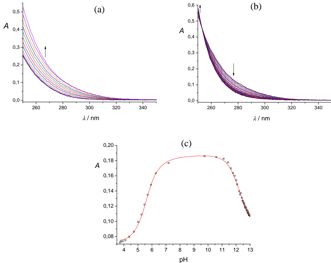
Slika 46. Spektrofotometrijsko-potenciometrijska titracija maleinske kiseline ( c = 4,88 \times 10^{-4} \text{ mol dm}^{-3} , V_0 = 40,35 \text{ cm}^3 ) s NaOH ( c = 5,00 \times 10^{-2} \text{ mol dm}^{-3} ) u metanolu; \theta = (25,0 \pm 0,1) \text{ }^\circ\text{C} , I_c = 0,01 \text{ mol dm}^{-3} ( \text{Et}_4\text{NCl} ), l = 1 \text{ cm} . a) pH-područje od 3,71 do 7,18; b) pH-područje od 7,18 do 13,04; c) ovisnost apsorbancije pri 270 nm o pH-vrijednosti otopine; \square eksperimentalne vrijednosti, - izračunane vrijednosti.
