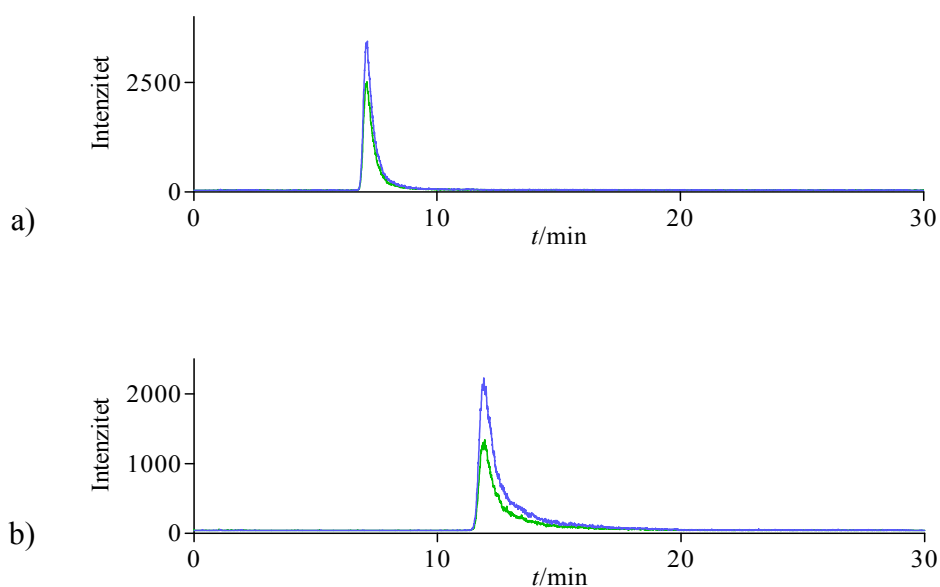
Slika 21. Kromatogrami višestrukih tranzicijskih reakcija [M]^+ \rightarrow 124 (plavo) i [M]^+ \rightarrow 107 (zeleno) NMP derivata masnih kiselina na koloni Hypersil Gold: a) c(\text{C}19:0) = 4,7 \cdot 10^{-5} \text{ mol L}^{-1} , b) c(\text{C}22:0) = 3,8 \cdot 10^{-5} \text{ mol L}^{-1} . NMP derivati masnih kiselina eluirani su upotrebom gradijenta mobilne faze prema Tablici 13.
