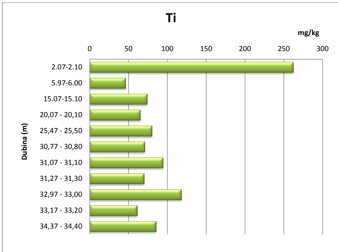
Slika 58. Koncentracija titana
