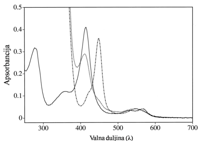
Slika 3. CYP119 iz Solfobus solfataricus . Puna linija: slobodni hemoprotein, Točkasta linija: hemoprotein reduciran ditionitom, Puna – istočkana linija: Hem – CO kompleks (Preuzeto iz Koo i sur., 2000).
