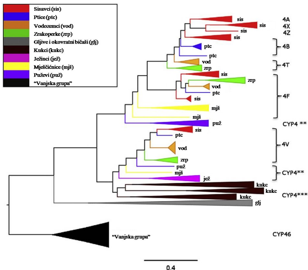
Slika 9. Filogenetska analiza citokroma P450 obitelji 4. Prikaz evolucijskih odnosa između CYP4 podobitelji beskranježnjaka i kralježnjaka. Grane koje uključuju cyp4 gene koji nisu dodijeljeni niti jednoj podobitelji označeni su CYP**. cyp4 geni Drosophila melanogaster koji predstavljaju 10 CYP4 podobitelji kukaca označeni su CYP*** (Preuzeto iz Kirischian i Wilson, 2012).
