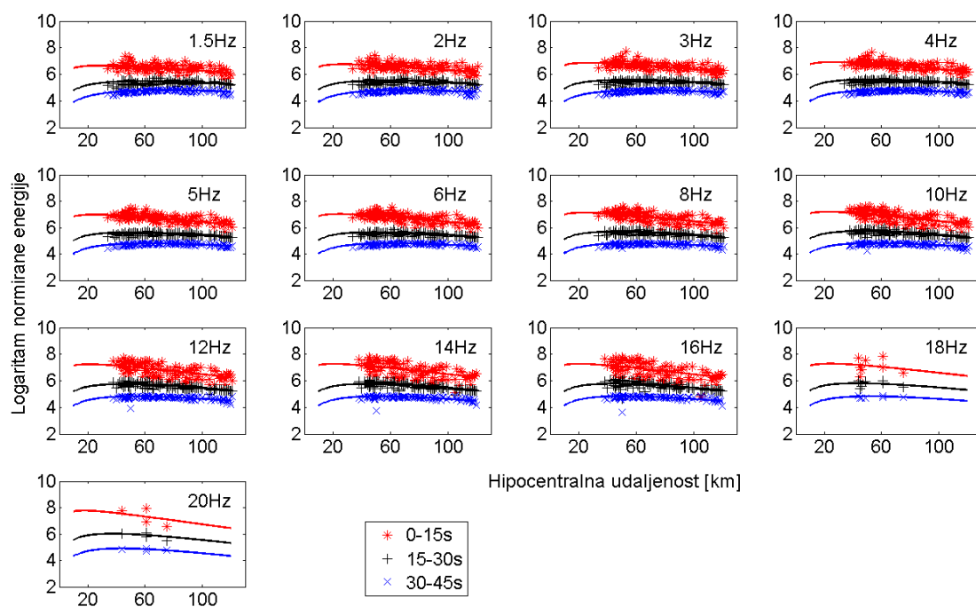
Slika A.3 Rezultati za postaju SLNJ. Izmjerene energije seizmograma, u tri vremenska prozora: 0–15 s (*), 15–30 s (+), 30–45 s (x), zajedno s teorijskim krivuljama energije koje predstavljaju najbolju prilagodbu mjerenjima, u ovisnosti o hipocentralnoj udaljenosti.
