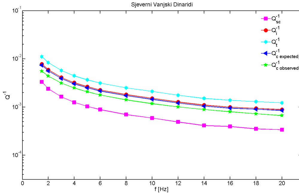
Slika 4.7 Q^{-1} -faktori dobiveni MLTWA metodom: faktor atenuacije raspršenja Q_{sc}^{-1} , intrinzične Q_i^{-1} i ukupne atenuacije Q_t^{-1} , očekivani Q_c^{-1} -faktor Q_c^{-1} \text{ expected} te mjereni Q_c^{-1} \text{ observed} preuzet iz Dasović (2015).
