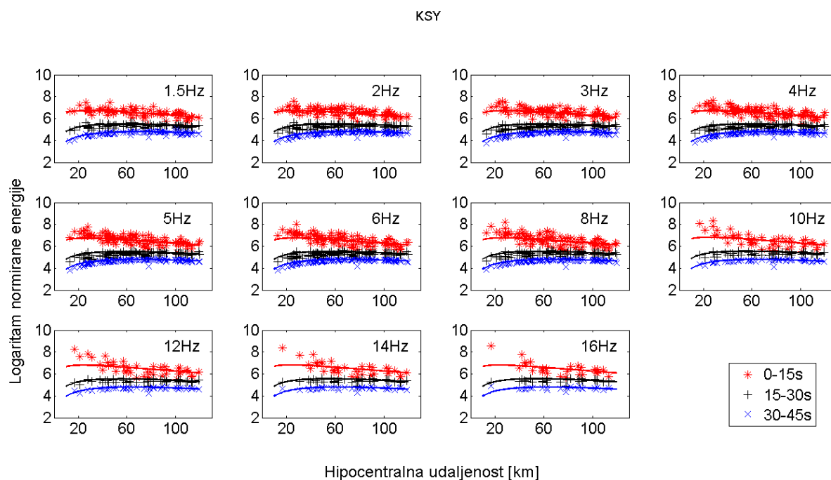
Slika 3.4 Izmjerene energije seizmograma postaje KSY u tri vremenska prozora: 0 – 15 s(*), 15 – 30 s(+), 30 – 45 s(×), zajedno s teorijskim krivuljama energije koje predstavljaju najbolju prilagodbu mjerenjima, u ovisnosti o hipocentralnoj udaljenosti.
