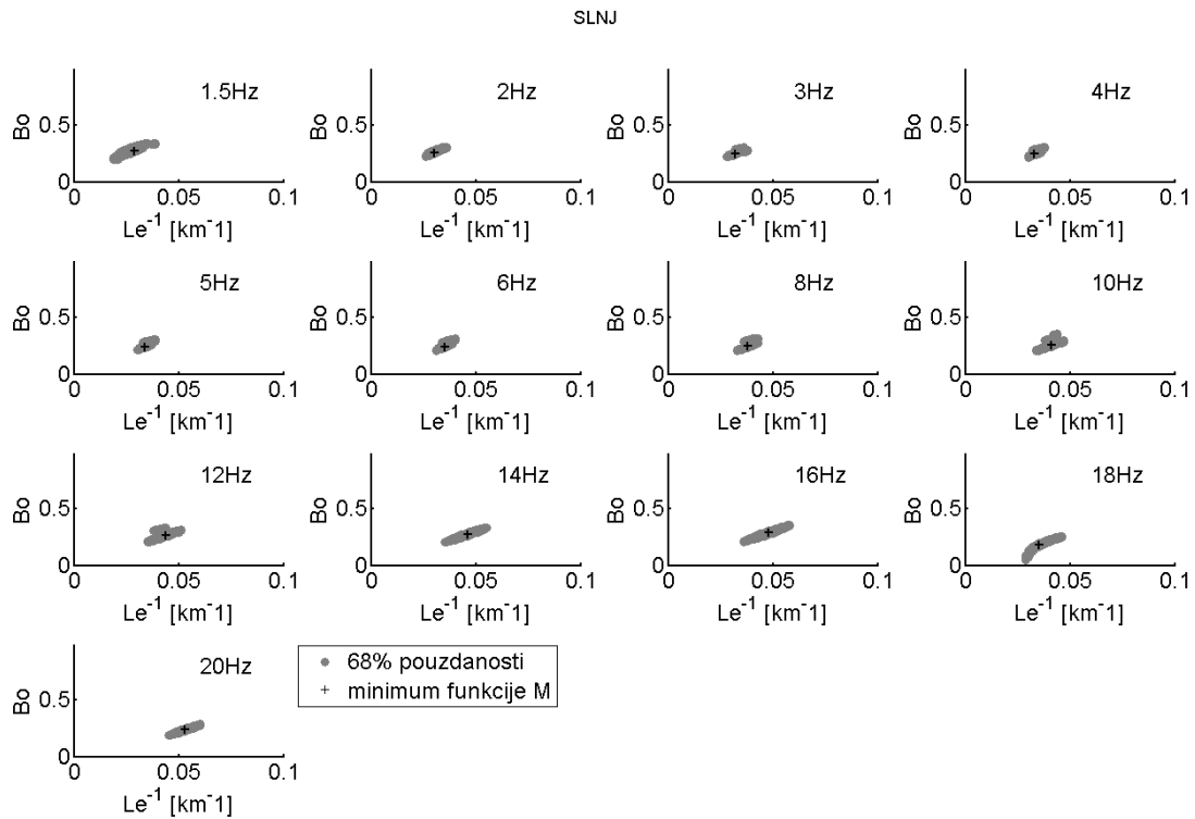
Slika A.9 Rezultati za postaju SLNJ. Parovi B_0 i Le^{-1} koji predstavljaju najbolju prilagodbu teorijske energije mjerenoj (+), po frekvencijama, te procjena intervala njihovih pogreški, koje odgovaraju području 68% pouzdanosti F-distribucije (sivo područje).
