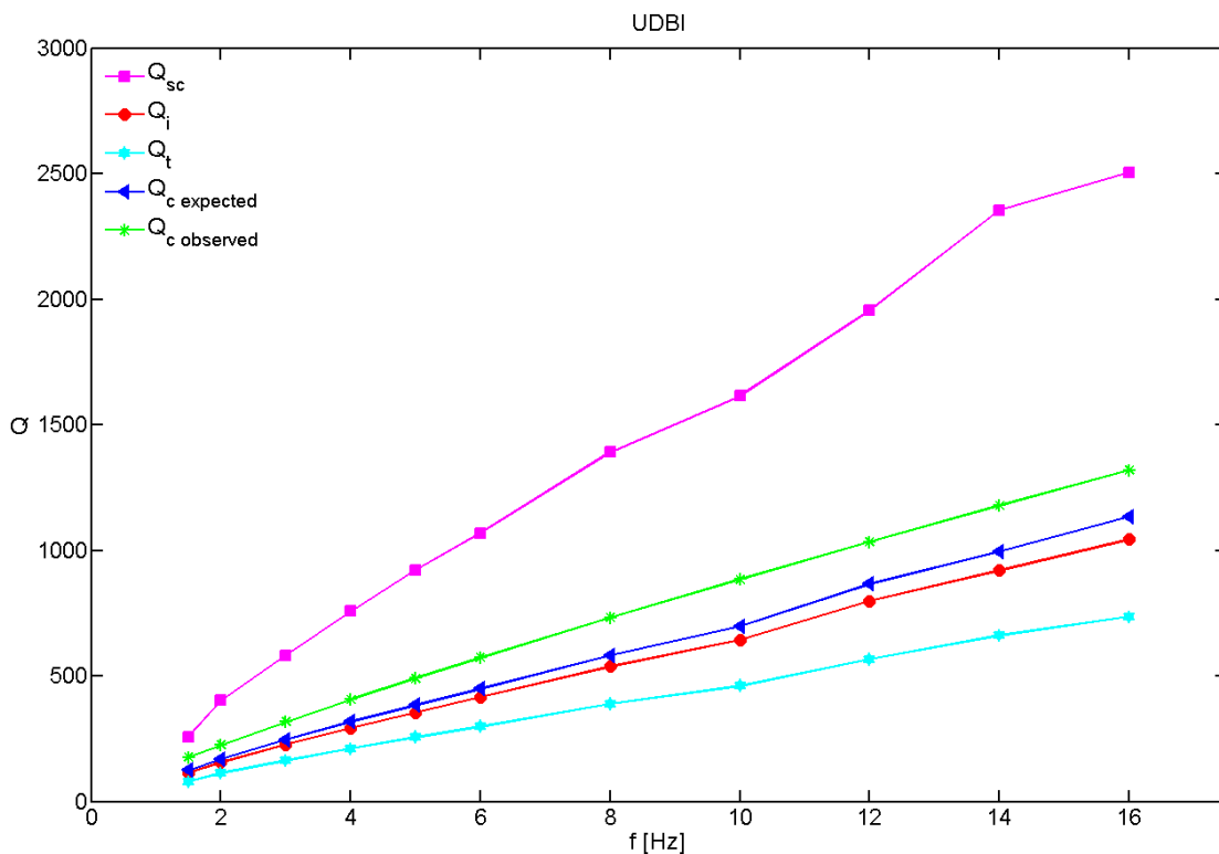
Slika A.20 Rezultati za postaju UDBI. Q -faktori u ovisnosti o frekvenciji dobiveni MLTWA metodom te mjereni Q_c observed preuzet iz Dasović (2015).
