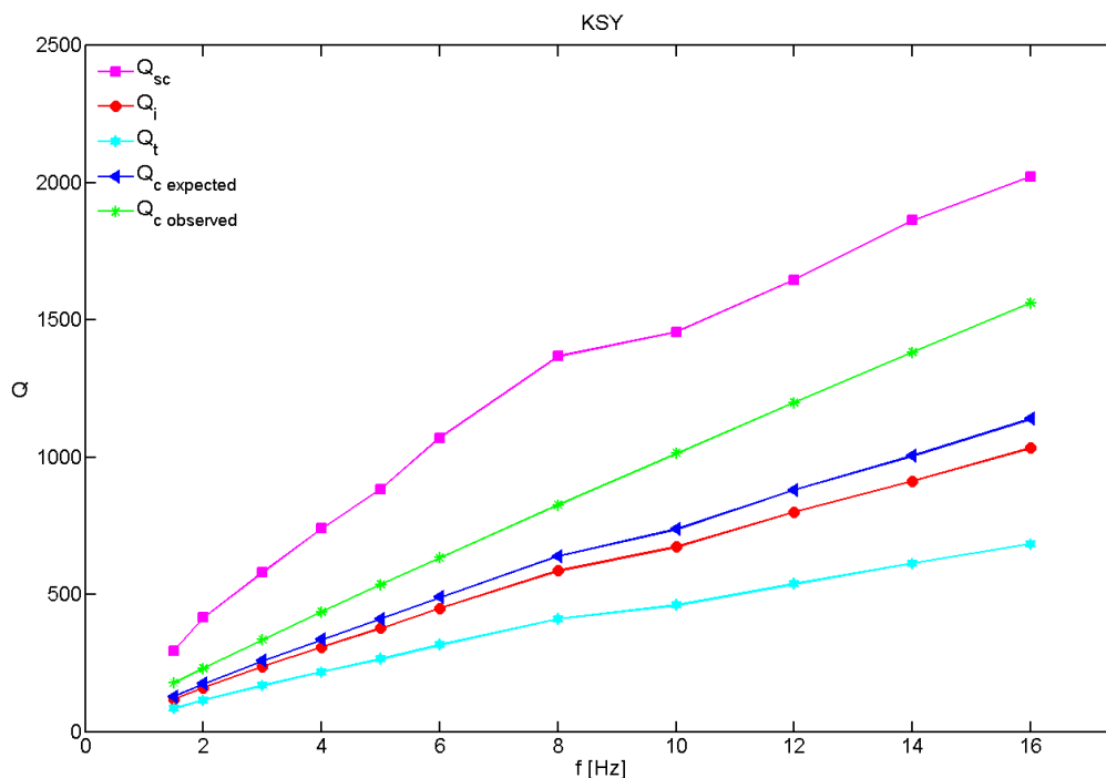
Slika 4.2 Q -faktori dobiveni MLTWA metodom: faktor dobrote raspršenja Q_{sc} , intrinzični Q_i i inverz ukupne atenuacije Q_t , očekivani Q_c -faktor Q_c \text{ expected} te mjereni Q_c \text{ observed} preuzet iz Dasović (2015). Rezultati za postaju KSY.
