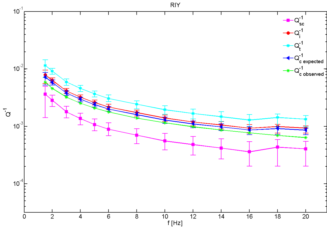
Slika A.17 Rezultati za postaju RIY. Q^{-1} -faktori u ovisnosti o frekvenciji dobiveni MLTWA metodom te mjereni Q_c^{-1} \text{ observed} preuzet iz Dasović (2015). Prikazane su i pripadajuće standardne devijacije dobivene za parove Le^{-1} i B_0 područja 68% pouzdanosti F-distribucije.
