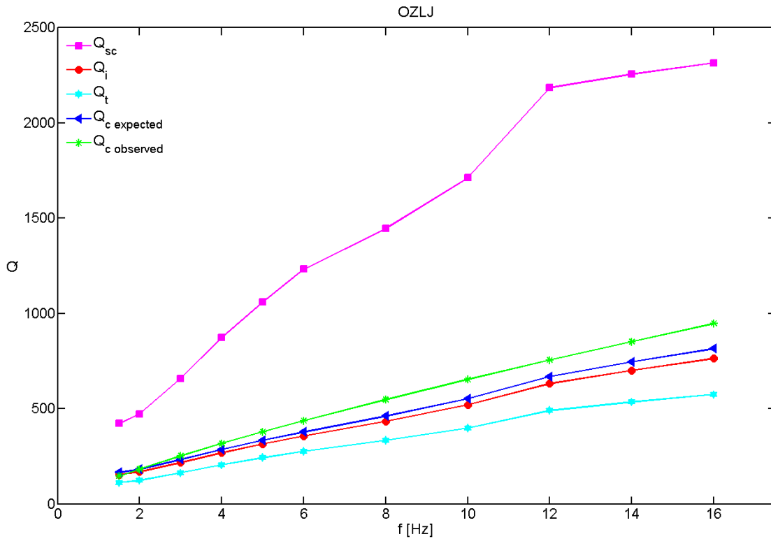
Slika A.19 Rezultati za postaju OZLJ. Q -faktori u ovisnosti o frekvenciji dobiveni MLTWA metodom te mjereni Q_c observed preuzet iz Dasović (2015).
