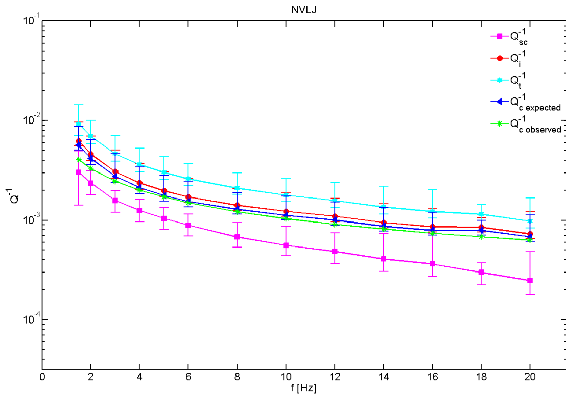
Slika A.16 Rezultati za postaju NVLJ. Q^{-1} -faktori u ovisnosti o frekvenciji dobiveni MLTWA metodom te mjereni Q_c^{-1} preuzet iz Dasović (2015). Prikazane su i pripadajuće standardne devijacije dobivene za parove Le^{-1} i B_0 područja 68% pouzdanosti F-distribucije.
