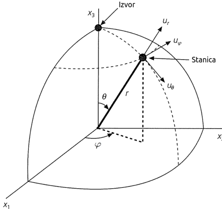
Slika 2.1 Sferni koordinatni sustav za normalne modove. Izvor potresa nalazi se u polu, tako da u položaju prijmnika radijalna komponenta pomaka u_r je vertikalna, u_\theta se nalazi u horizontalnom položaju u vertikalnoj ravnini koja sadrži i izvor i prijmnik, dok je pomak u_\varphi transverzalan na tu ravninu. Preuzeto iz Sten i Wyssession (2003).
