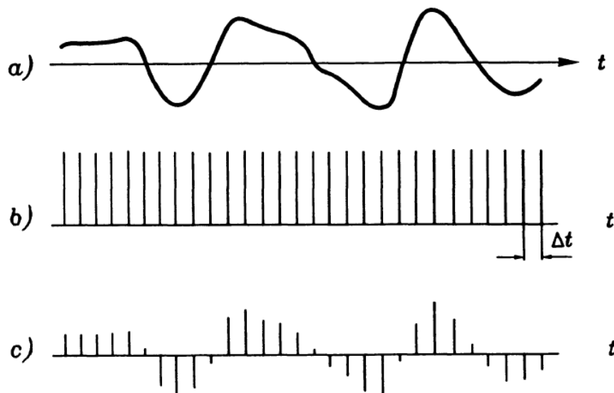
Slika 2.4 Prikaz uzorkovanja kontinuirane funkcije x(t) (a), gdje je funkcija uzorkovanja niz Delta funkcija \delta(t - j\Delta t) (b), a rezultat je funkcija x_s(t) (c). Preuzeto iz Butkus (2000).
