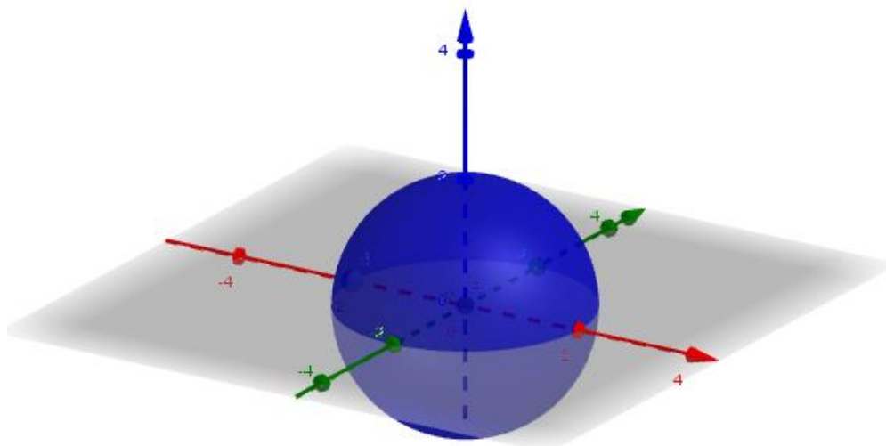
Slika 2.3.2 Sfera x^2 + y^2 + z^2 = 4
