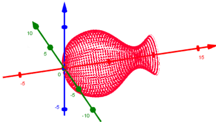
Slika 2.3.6 Rotacija polinomne krivulje oko osi x
