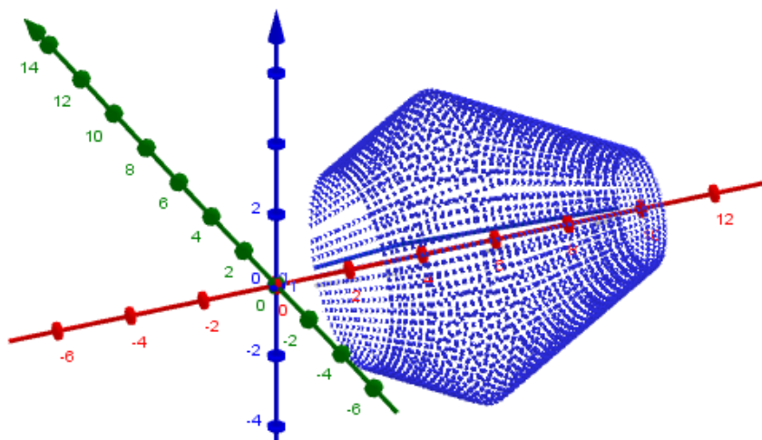
Slika 2.3.5 Rotacija krivulje g(x) = -\frac{1}{2}|x - 5| + 4, x \in [2, 10] oko osi x
