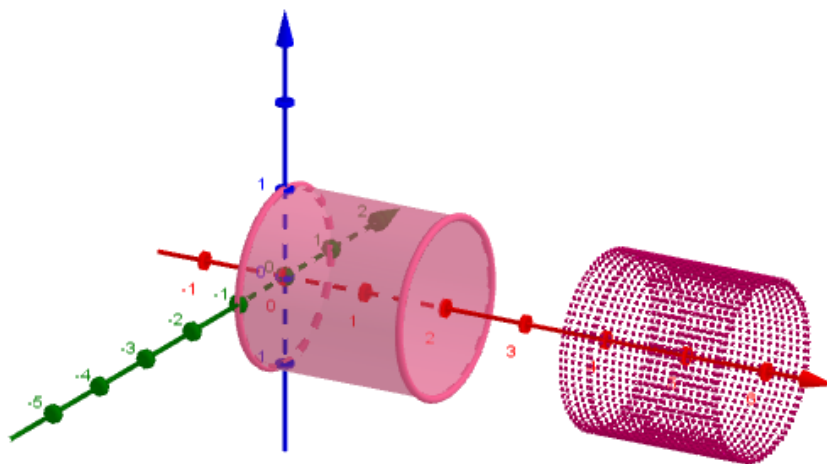
Slika 2.3.4 Valjak konstruiran alatom Valjak i valjak konstruiran rotacijom
