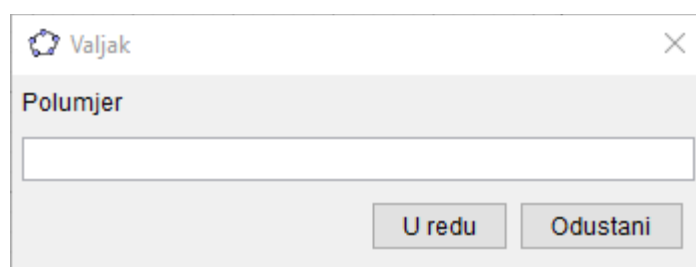
Slika 2.3.3 Dijaloški okvir Valjak
