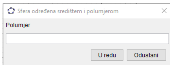
Slika 2.3.1 Dijaloški okvir Sfera određena središtem i polumjerom
