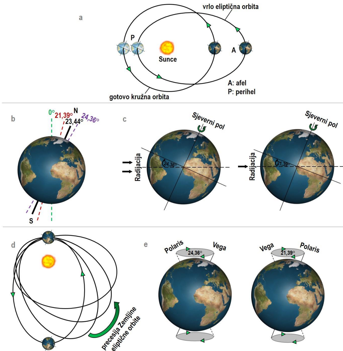
Slika 3 Milankovićeve ciklusi: (A) ekscentricitet Zemljine putanje oko Sunca, (B), (C) promjena nagiba Zemljine osi, (D) precesija Zemljine eliptične orbite, (E) precesija Zemljine osi. Preuzeto i preuređeno prema http://gulfcoastcommentary.blogspot.hr/2013/11/what-causes-ice-ages.html , http://www.indiana.edu/~geol105/images/gaia_chapter_4/milankovitch.htm ; http://slideplayer.com/slide/6857046/
