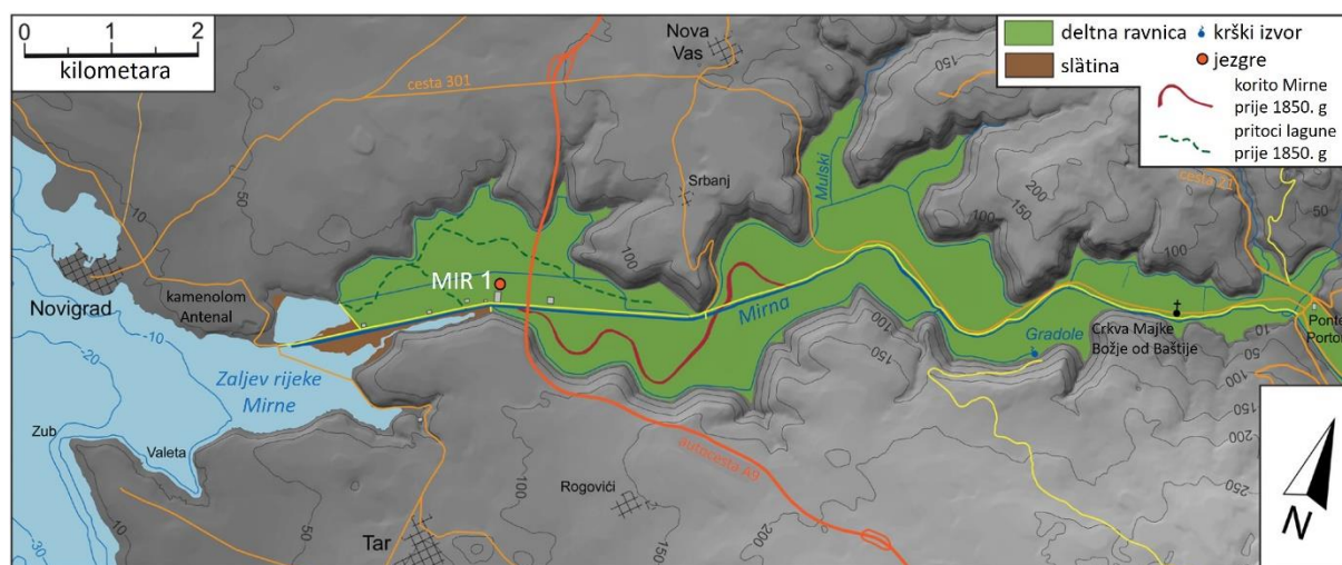
Slika 6 Uže područje deltna ravnice rijeke Mirne s označenim lokalitetom uzorkovanja. Preuzeto i preuređeno iz rada FELJA et al., 2015 i iz doktorske disertacije FELJA, 2017.
