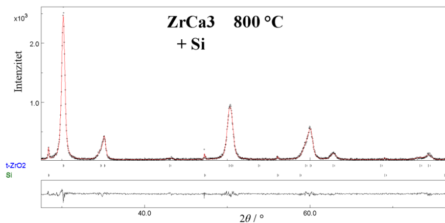
Slika D11. Rezultat Rietveldovog utočnjavanja difraktograma uzorka \text{ZrCa}_3 žarenog na 800\text{ °C} . Razlika izračunatog i dobivenog difraktograma prikazana je u donjem pravokutniku.
