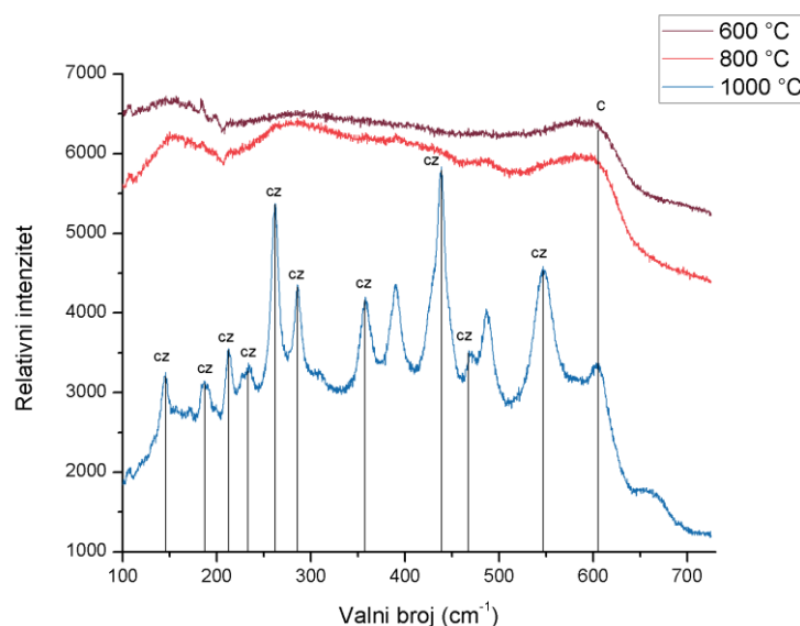
Slika 4.13. Ramanovi spektri uzorka ZrCa30 žarenog na temperaturama od 600, 800 i 1000 °C. Oznakom c označena je vrpca koja odgovara vrpca c\text{-ZrO}_2 polimorfa, a oznakom cz vrpce koje odgovaraju vrpca kalcijeva cirkonata.
