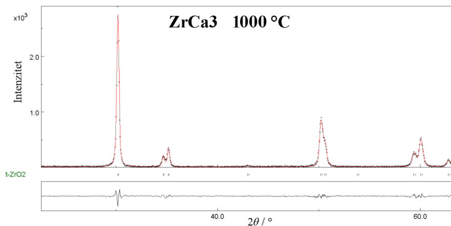
Slika D12. Rezultat Rietveldovog utočnjavanja difraktograma uzorka \text{ZrCa}_3 žarenog na 1000\text{ °C} . Razlika izračunatog i dobivenog difraktograma prikazana je u donjem pravokutniku.
