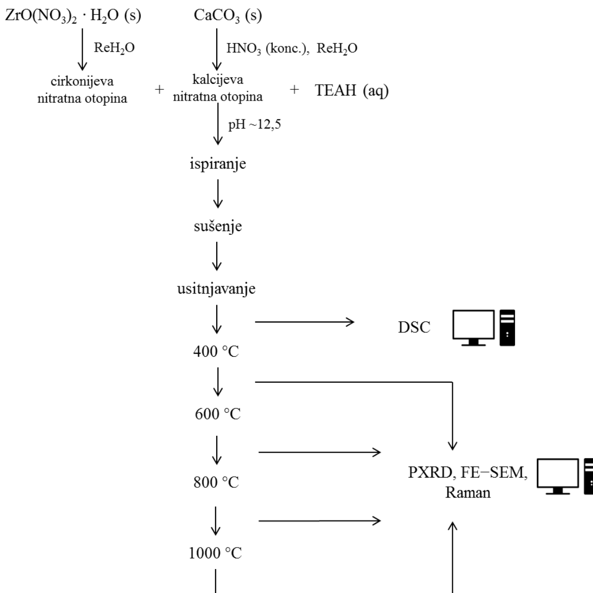
Slika 3.2. Shema metode I za sintezu i katarakterizaciju čvrstih otopina \text{ZrO}_2\text{-CaO} .
