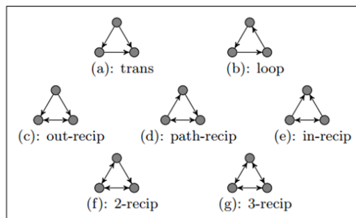
Slika 2.2: Usmjereni trokuti
