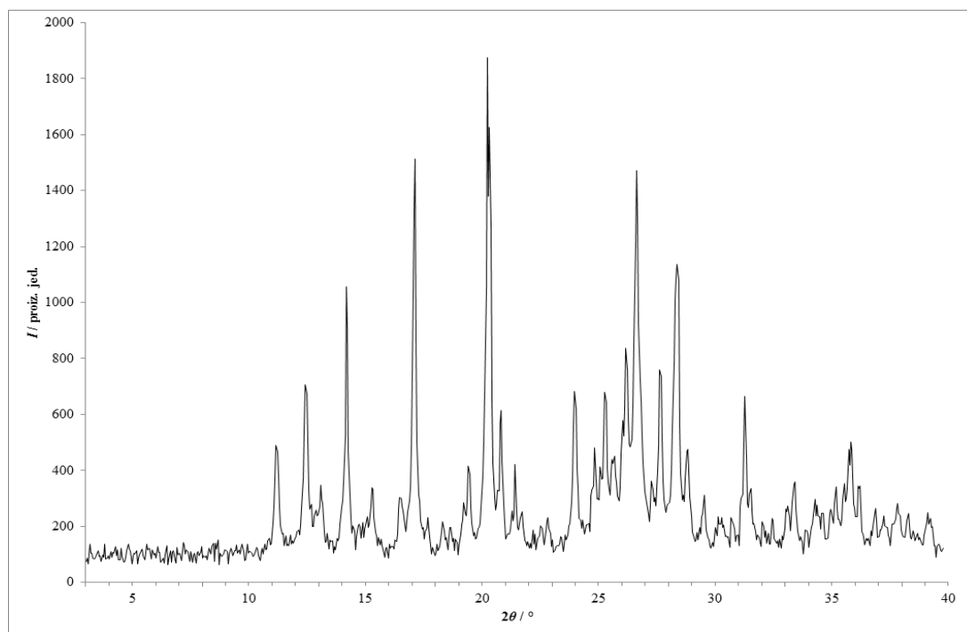
Slika 97 – Rentgenski difraktogram praškastog uzorka dobivenog kristalizacijom iz otopine lam i fru u etanolu.
