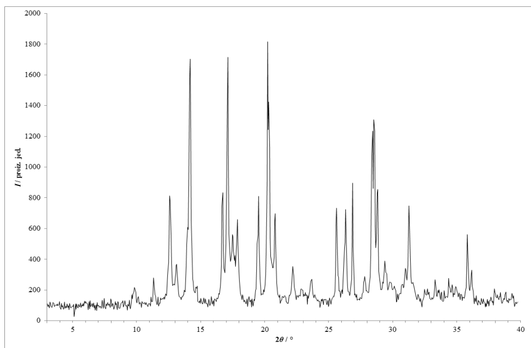
Slika 98 – Rentgenski difraktogram praškastog uzorka dobivenog kristalizacijom iz otopine lam i fru u etil-acetatu.
