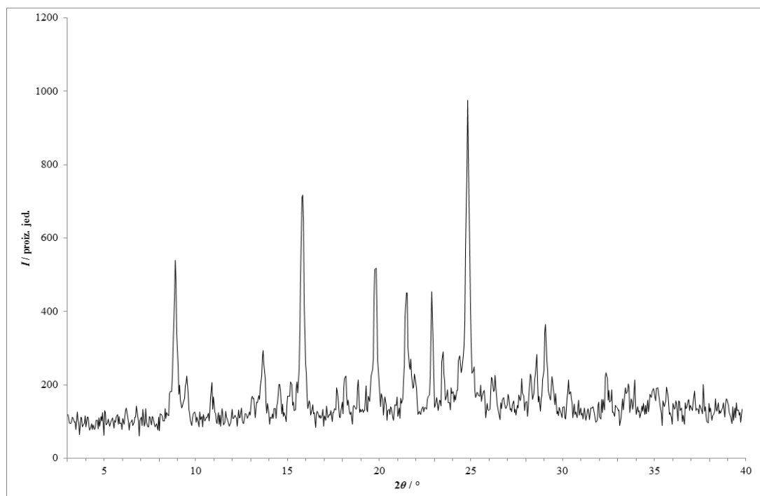
Slika 109 – Rentgenski difraktogram praškastog uzorka dobivenog ručnom mehanokemijskom sintezom fizičke smjese lam i van s dodatkom katalitičke količine acetona.
