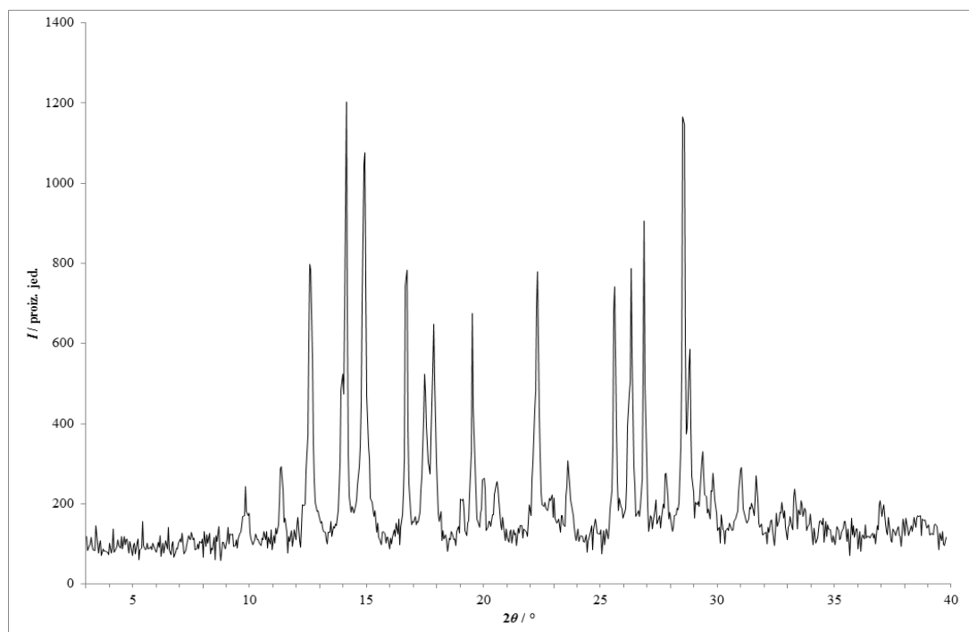
Slika 143 – Rentgenski difraktogram praškastog uzorka dobivenog ručnom mehanokemijskom sintezom fizičke smjese lam i nia s dodatkom katalitičke količine acetona.
