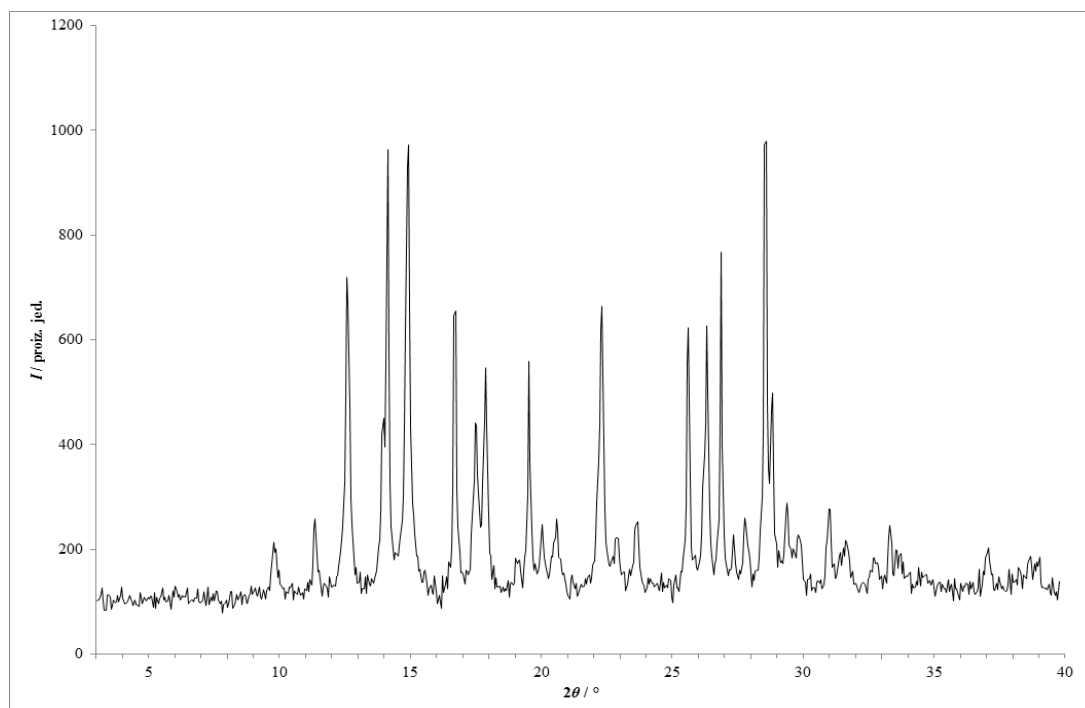
Slika 153 – Rentgenski difraktogram praškastog uzorka dobivenog ručnom mehanokemijskom sintezom fizičke smjese lam i nia s dodatkom katalitičke količine metanola.
