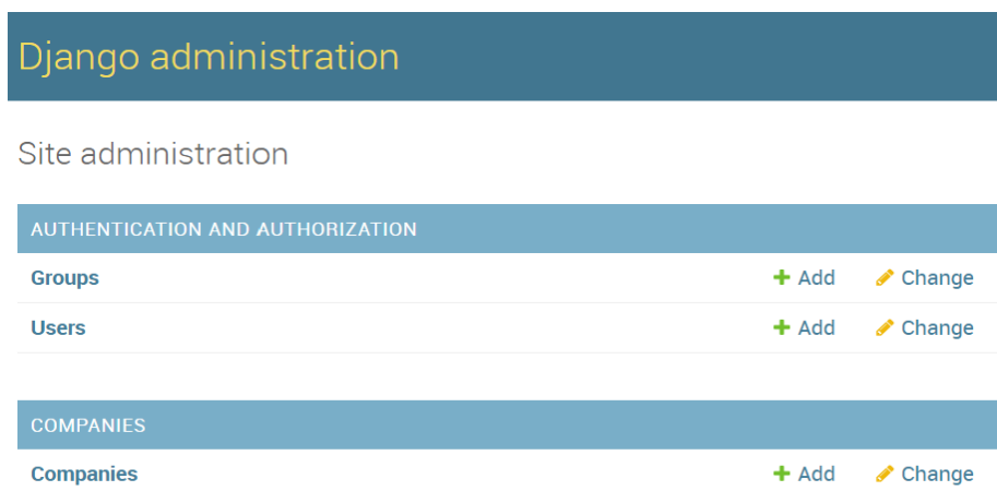
Slika 2.1: Django administracija
