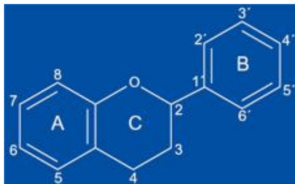
Slika 1.1. Opća struktura kemijskog spoja koji pripada skupini flavonoidnih pigmenata.
