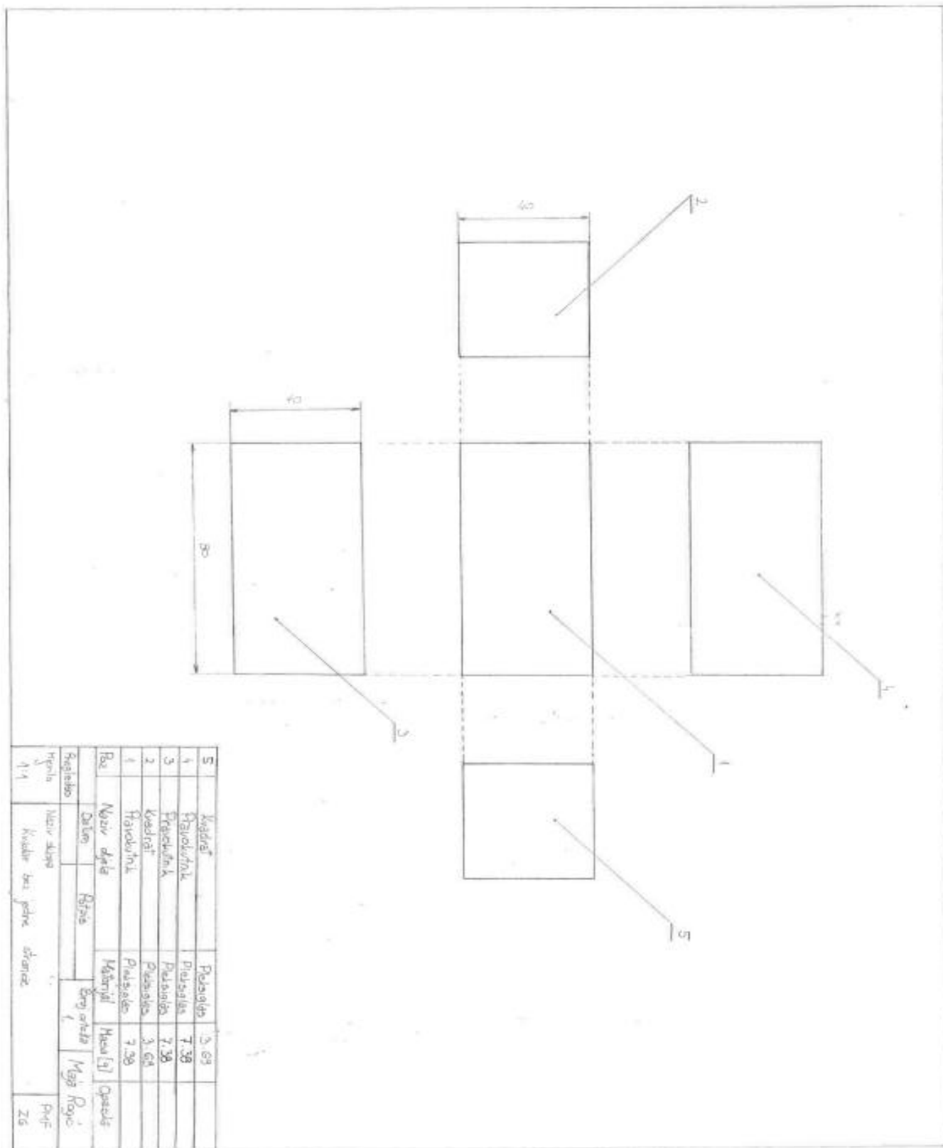
Slika 1. Montažni crtež kvadra.
