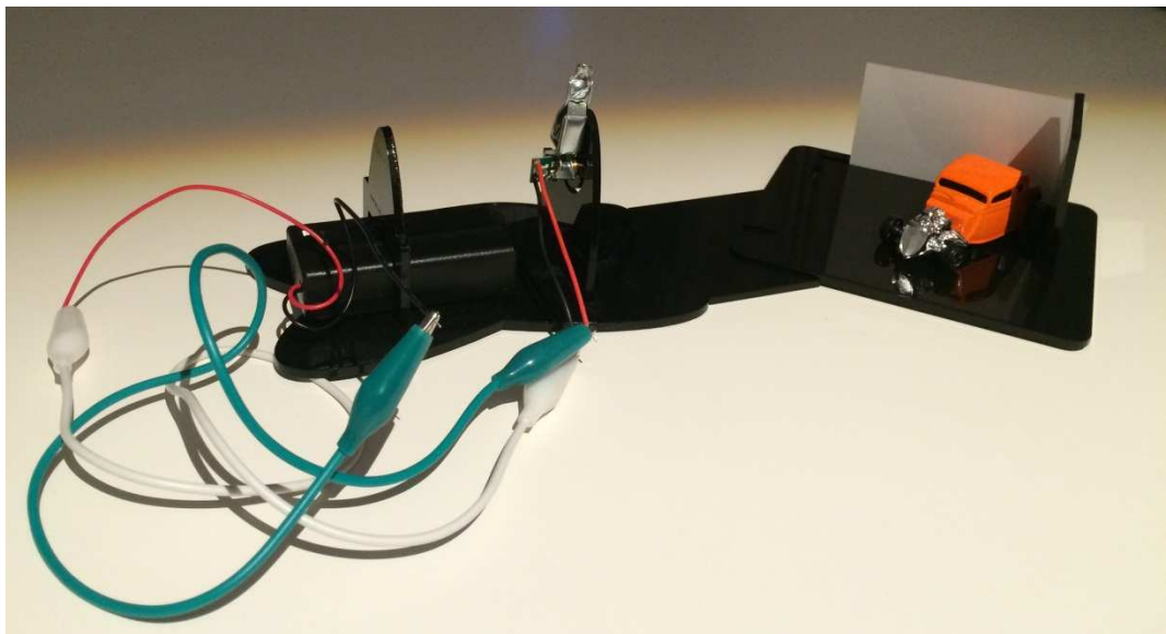
Slika 4.5.9 Postav holograma
