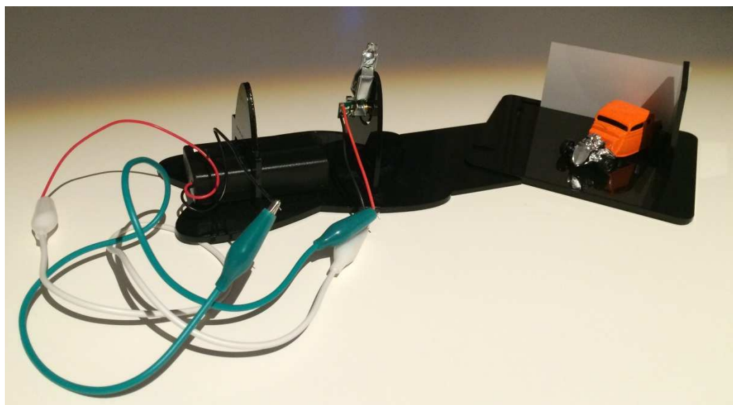
Slika 4.5.9 Postav holograma
