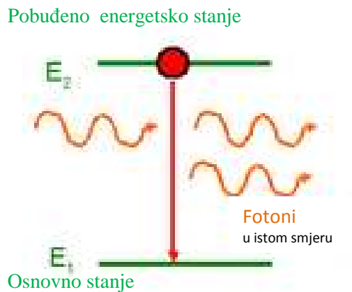
Slika 2.3.3 Stimulirana emisija [18]
