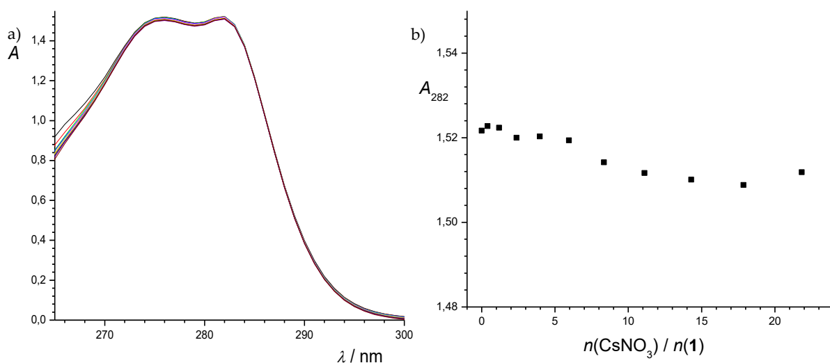
Slika 29: a) Spektrofotometrijska titracija spoja 1 ( c = 4,95 \times 10^{-4} \text{ mol dm}^{-3} , V_0 = 2,0 \text{ cm}^3 ) s cezijevim nitratom ( c = 1,95 \times 10^{-2} \text{ mol dm}^{-3} ) u N,N -dimetilformamidu. b) Ovisnost apsorbancije o množinskom omjeru n(\text{CsNO}_3)/n(\mathbf{1}) . Vrijednosti su korigirane za razrjeđenje i za apsorpciju nitratne skupine. l = 1 \text{ cm} ; \vartheta = (25,0 \pm 0,1) \text{ }^\circ\text{C} ; ■ eksperimentalne vrijednosti.
