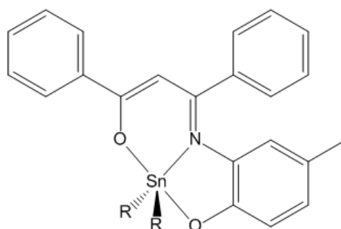
Slika 12. Struktura [R_2SnL] , L = 3-(2\text{-hidroksi-5-metilfenilamino})\text{-1,3-difenilprop-2-en-1-on} , R = \text{metil, fenil} .
