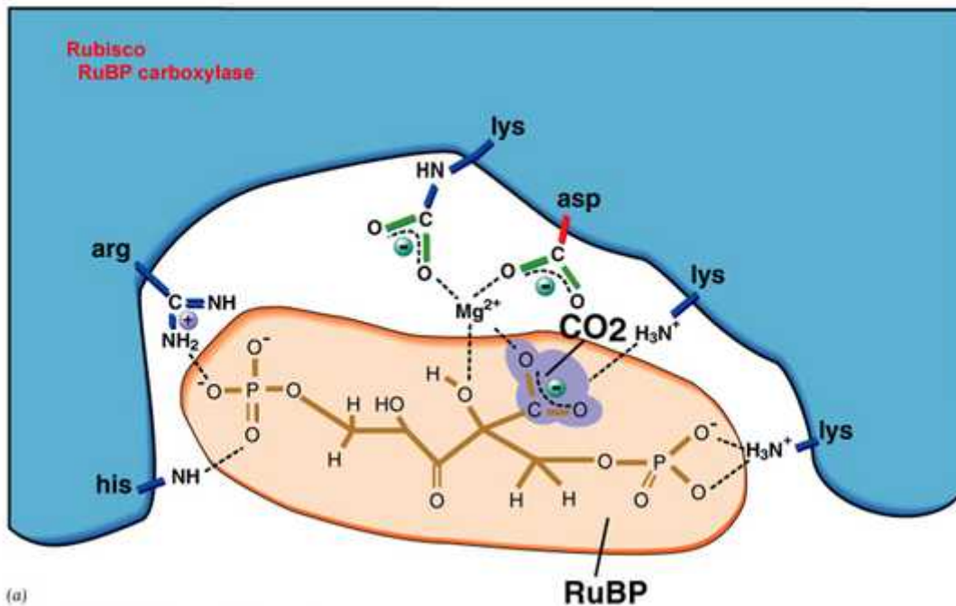
Slika 5. \epsilon -amino skupina lizina-334 uz \text{Mg}^{2+} stabilizira prijelazno stanje. Preuzeto i prilagođeno www.chemwiki.ucdavis.edu/Wikitexts/UC_Davis/UCD_Chem_124A%3A_Berben/Ribulose_1,5-bisphosphate_carboxylase_(rubisco)/Rubisco_1
