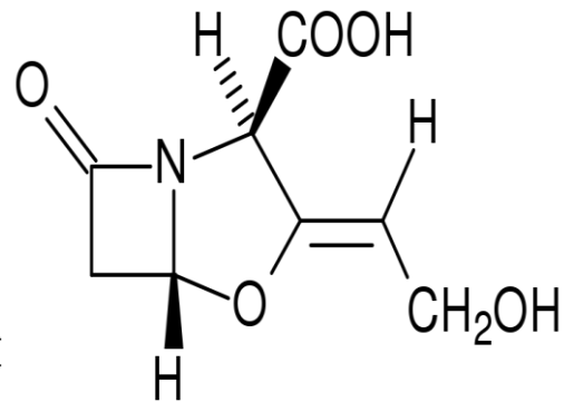
Slika 3. A Opća struktura penicilina, B Struktura klavulanske kiseline
