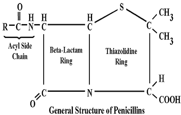
Slika 3. A Opća struktura penicilina, B Struktura klavulanske kiseline
