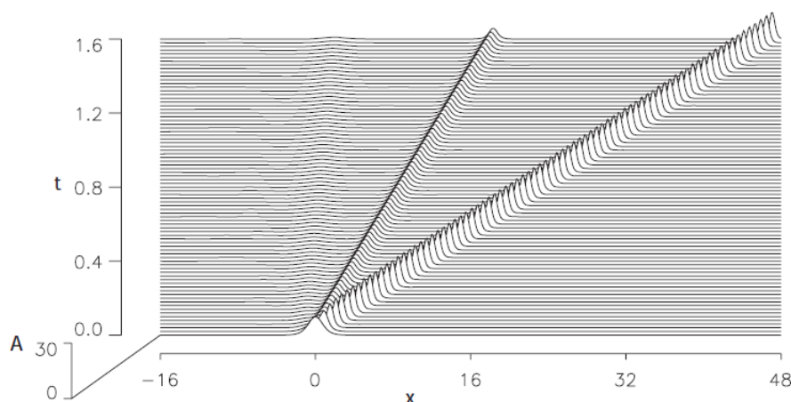
Slika 4. Generiranje tri solitona od lokalnih inicijalnih uvjeta u KdV jednadžbi (1.2)
