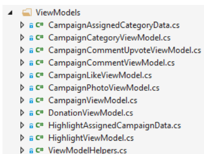
Slika 2.10: Direktorij ViewModels
