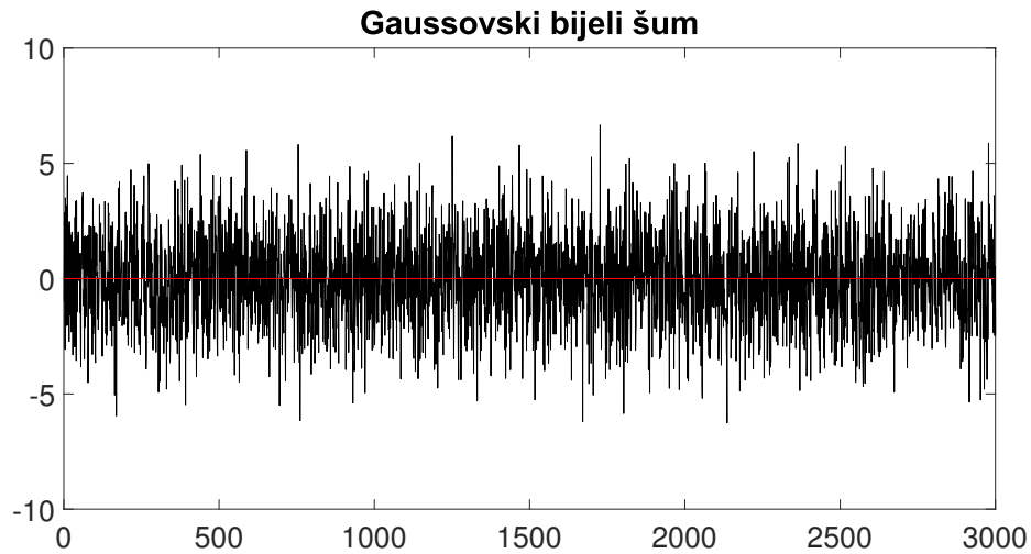
Slika 5.1: Gaussovski bijeli šum \{\xi_n\} s varijancom \sigma^2 = 4
