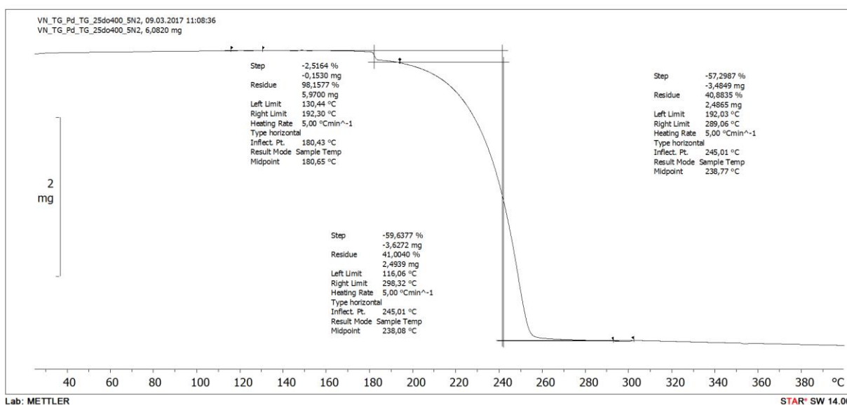
Slika D36. TG krivulja čistog Pd(acac) 2 .
