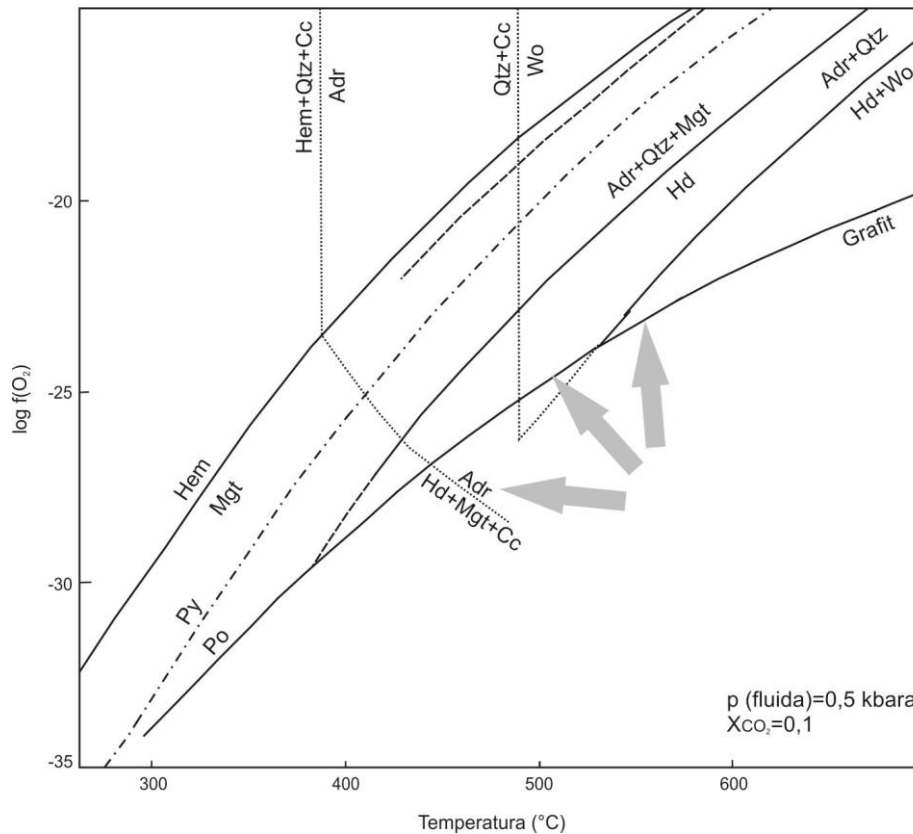
Slika 6.6. Temperatura-log f(\text{O}_2) dijagram s prikazanim poljima stabilnosti za Fe-skarske minerale (Meinert, 1982). Dijagram vrijedi za pritiske fluida od 0,5 kbara i molarni udio \text{CO}_2 od 0,1.
