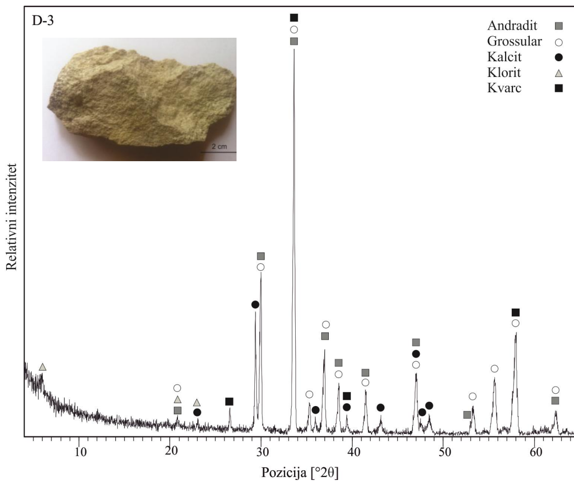
Slika II. Rentgenogram uzorka D-3.
