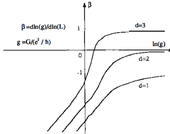
Slika 3.2: Dimenzionalna ovisnost funkcije \beta(g) = d \ln(g)/d \ln L kao funkcija vodnosti g . Za d = 1, 2 \beta(g) je strogo negativna i asimptotski teži nuli za veliki g i d = 2 . To indicira da nema metal-izolator za d = 1, 2 te da su u niskim dimenzijama stanja uvijek lokalizirana. U d = 3 , \beta(g) siječe os \beta(g) = 0 pa sukladno tome teorija predviđa i prijelaz između izolatorskog i metalnog stanja. Preuzeto iz [39].
