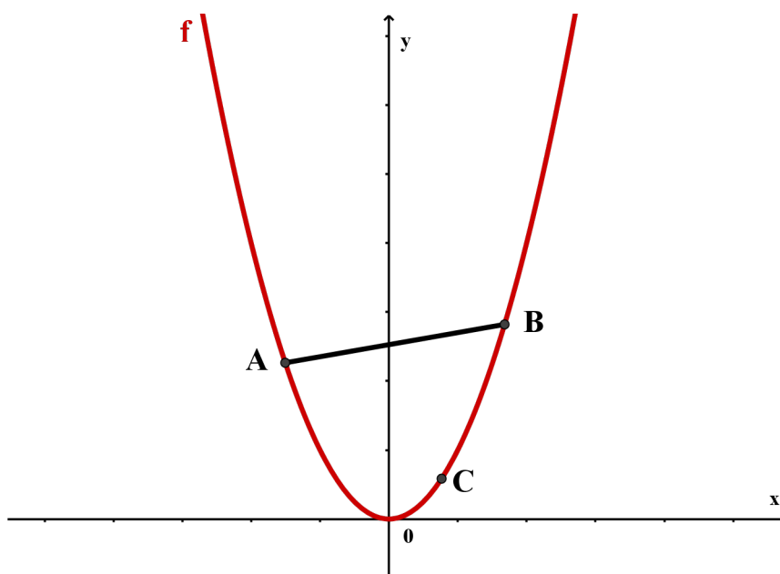
Slika 1.2: Konveksni graf
