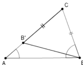
Slika 2.22: Dokaz Teorema 2.2.22 (1)
