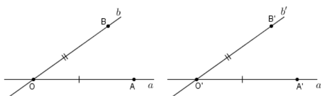
Slika 2.6: Dokaz Leme 2.1.12 (1)
