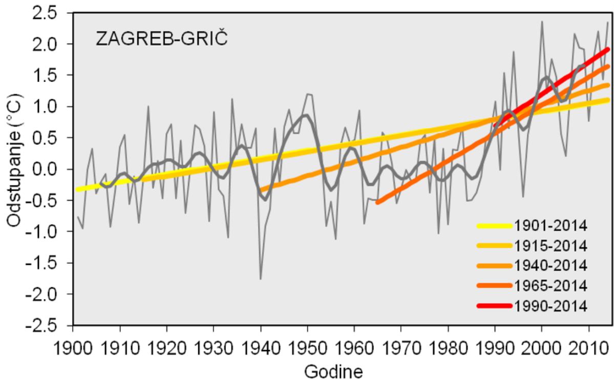
Sl. 2. Trendovi srednje temperature zraka u razdoblju 1901.-2014. Izvor: Ivančan-Picek, 2017
