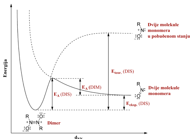
Slika 13. Dijagram prikazuje promjenu potencijalne energije tijekom konverzije trans -azodioksi dimera u dvije monomernne molekule C-nitrozo spoja, na način koji je predložio Lüttke. Na energijskom dijagramu d_{NN} predstavlja udaljenost između dva atoma dušika, E_A (DIS) energiju disocijacije dimerne molekule, E_A (DIM) energiju aktivacije za reakciju dimerizacije monomernih molekula, E_{teor.} (DIS) energiju disocijacije dimera koja zanemaruje doprinos elektronske reorganizacije, E_{eksp.} (DIS) energiju disocijacije dimera određene eksperimentalno.
