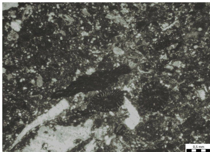
Slika 11 Bioklastični wackestone, SMF 9; uzorak Ld–2a.
