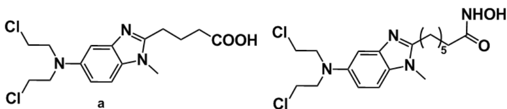
Slika 10. Bendamustin (a) i njegov analog 17
