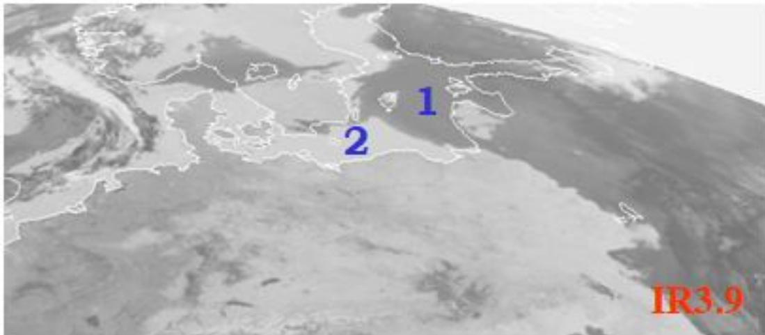
Slika 3.5: SEVIRI snimka Zemljine polutke, 24.04.2003. u kanalu IR3.9. (EUMETSAT - MSG Interpretation guide, 2018)
