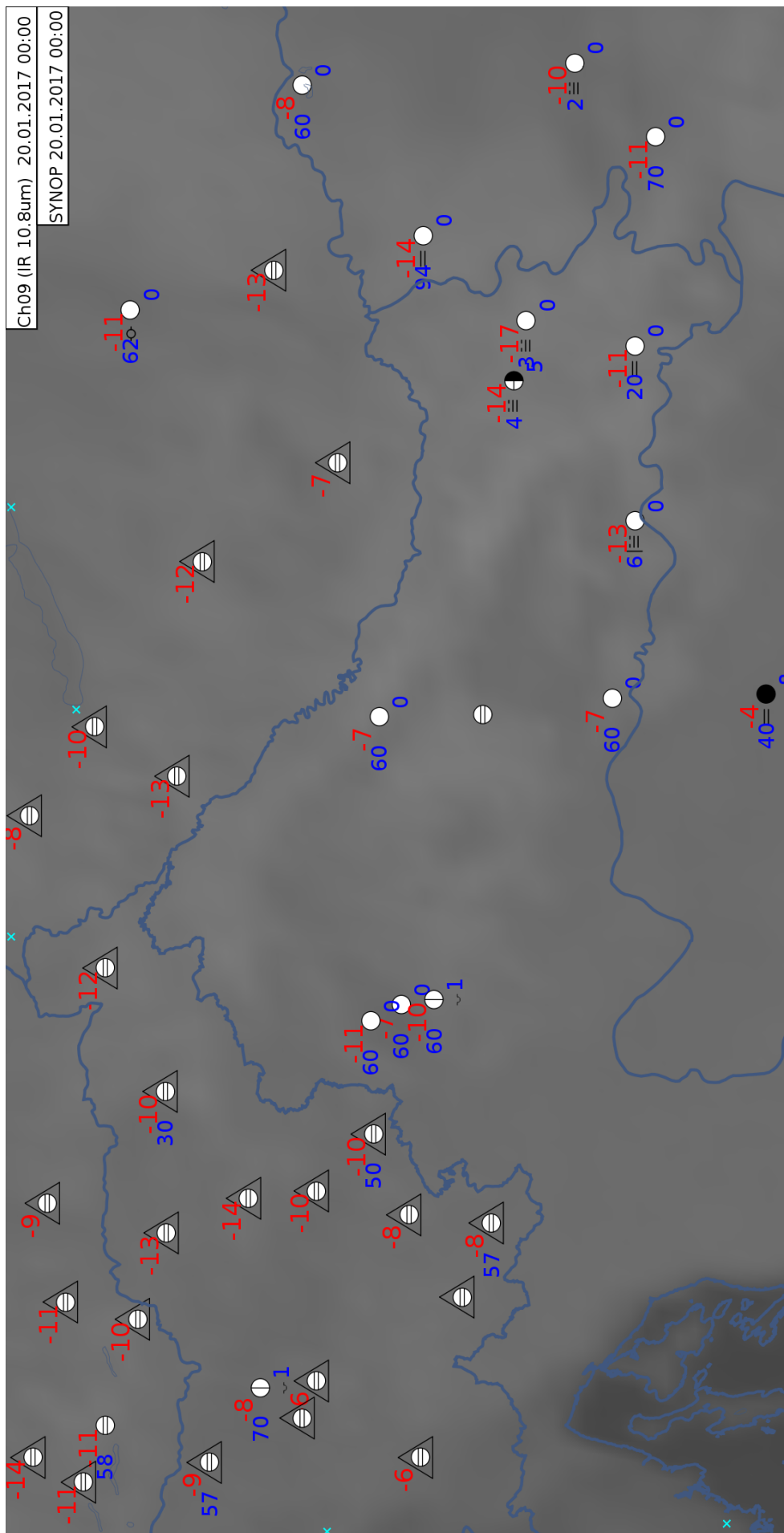
Slika 5.4: Sinopi i satelitska snimka u kanalu IR10.8 za 20.01.2017. u 00 UTC.
