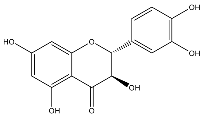
Slika 16: Struktura taksifolina
