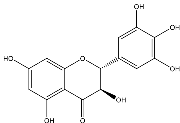
Slika 15: Struktura amelopsina
