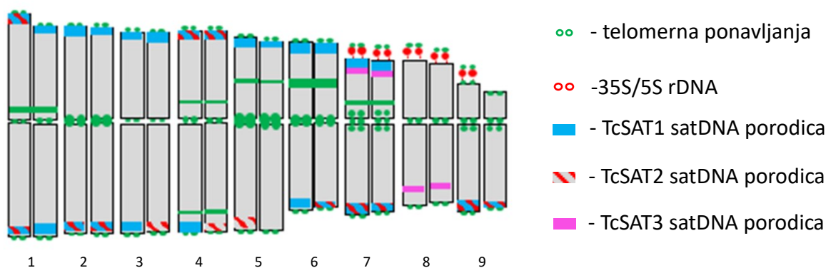
Slika 17. Idiogram vrste Tanacetum cinerariifolium . Na idiogramu su prikazani položaji: Arabidopsis -tipa telomernih ponavljajućih sekvenci, 35S/5S rDNA i satelitnih porodica TcSAT1, TcSAT2 i TcSAT3. Kromosomi su poredani po veličini i morfoloiji. Skala 10 \mu m
