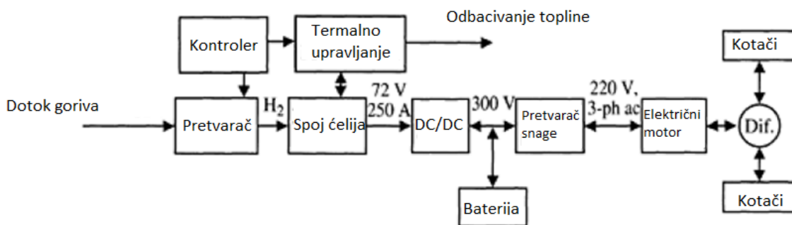
Slika 5: Shematski prikaz komponenti vozila na gorive ćelije[6]
