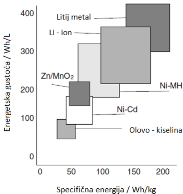
Slika 11: Prikaz domena vrijednosti energijske gustoće i specifične energije za različite tipove baterija [1]
