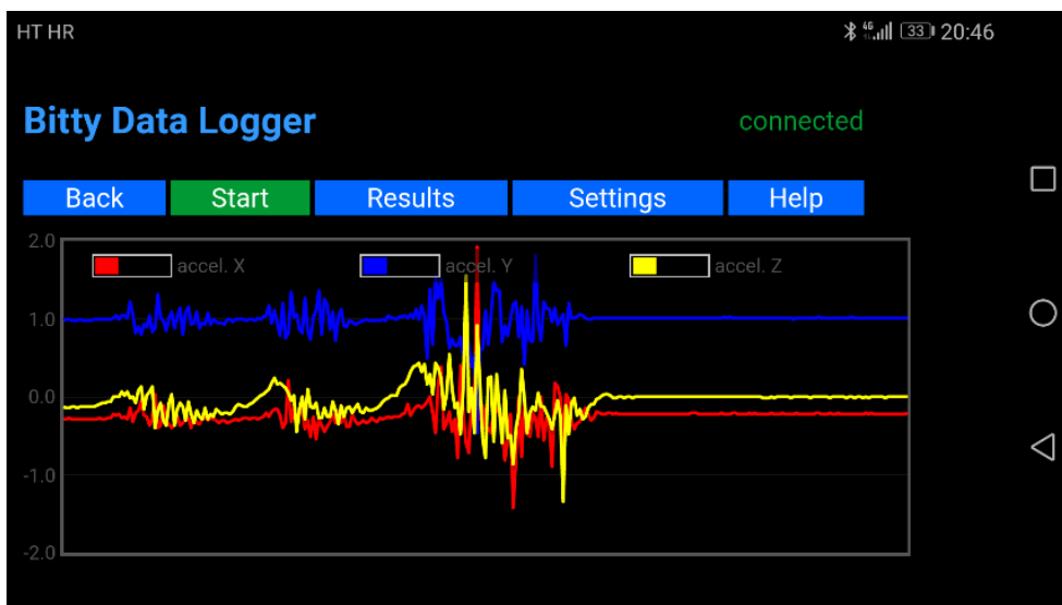
Slika 4.1.4. Grafički prikaz ovisnosti akceleracije o vremenu za slučaj kada djelujemo na tijelo silom koja nije stalna (povlačimo uže privezano za autić manjom ili većom silom).
