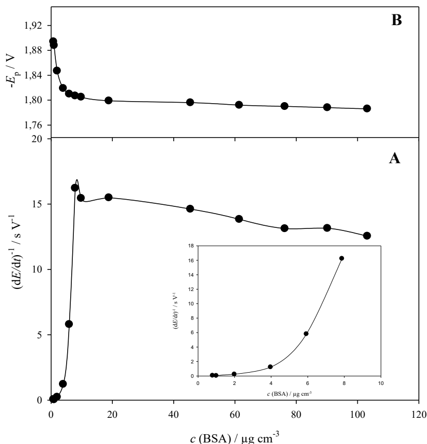
Slika 28. AdT CPS ovisnost visine (A) i položaja (B) pika H BSA o koncentraciji BSA u 0,05 \text{ mol dm}^{-3} fosfatnom puferu pH 7,05. Uvjeti mjerenja: E_a = -0,1 \text{ V} , I_{\text{str}} = -40 \mu\text{A} , t_a = 60\text{s} .
