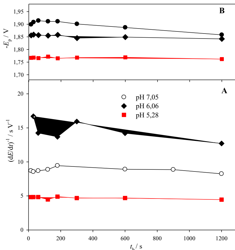
Slika 18. Stabilnost sloja kitozana ( c = 50 \times 10^{-6} \text{ g cm}^{-3} ) na živoj elektrodi u fosfatnom puferu pH 7,05, pH 6,06 i pH 5,28; uvjeti mjerenja: E_a = -0,1 \text{ V} , I_{\text{str}} = -20 \mu\text{A} (pH 7,05, pH 5,28) i -30 \mu\text{A} (pH 6,06), t_a = 60 \text{ s}
