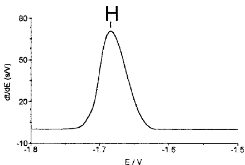
Slika 1. Pik H dobiven CPS analizom proteina vazopresina ( c = 1 \times 10^{-6} \text{ mol dm}^{-3} ) na HMDE u amonijakalnom puferu bez dodatka kobalta, pH 7,80, E_a 0,0 V, t_a 60 s, I_{str} = 20 \text{ } \mu\text{A} . Slika je preuzeta iz literaturnog izvora 28
