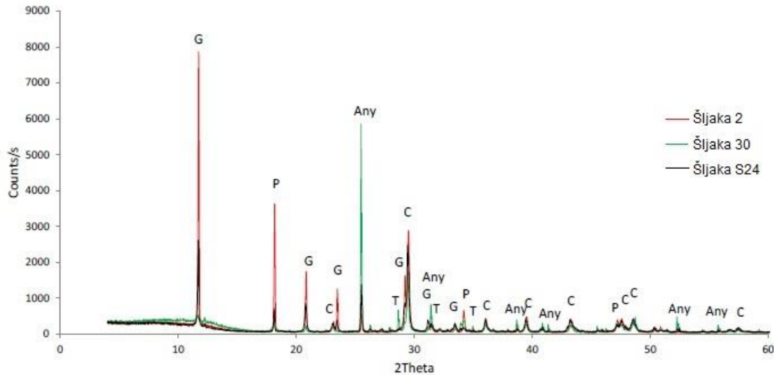
Slika 13. XRD difraktogram uzoraka šljake: Šljaka 2, Šljaka 30 i Šljaka S24. G-gips, Any-anhidrit, P-portlandit, C-kalcit i T-ternesit.
