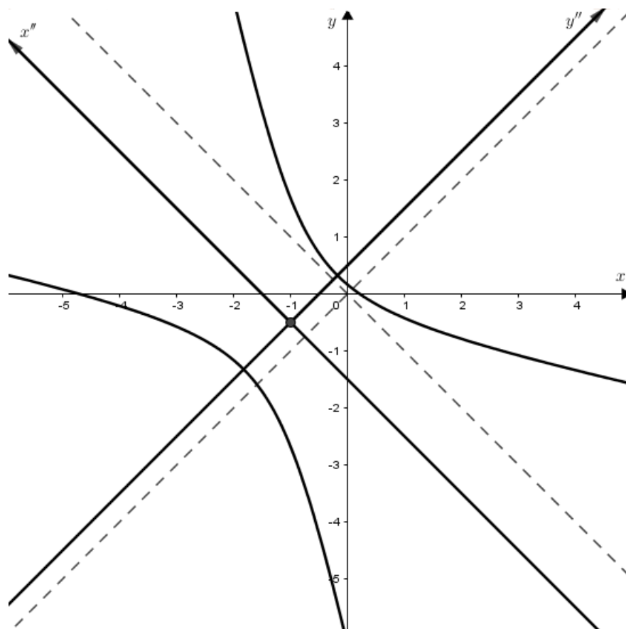
Slika 4.3: Dana hiperbola prikazana u koordinantnom sustavu xy
