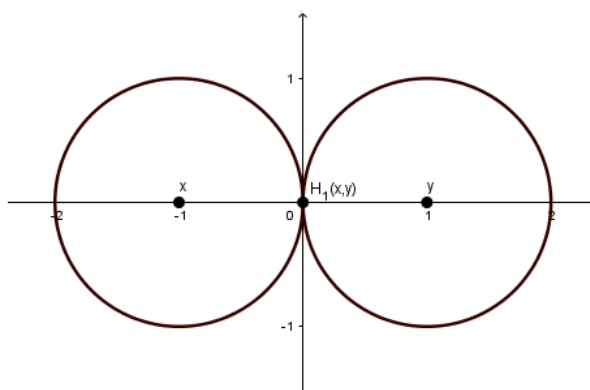
Slika 3.1: Centar para x, y je (0, 0)
