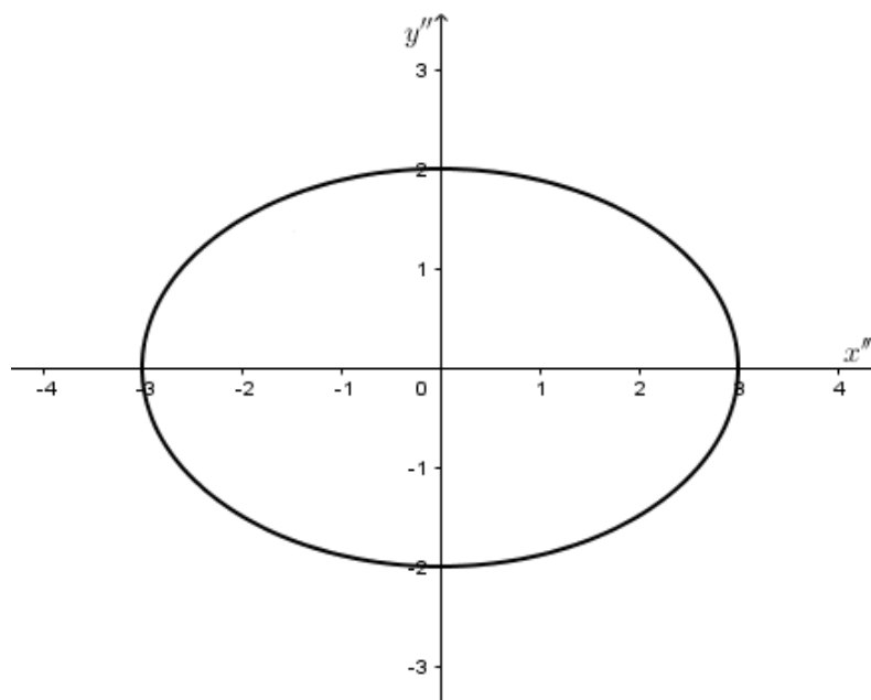
Slika 4.1: Dana elipsa prikazana u koordinatnom sustavu x''y''
