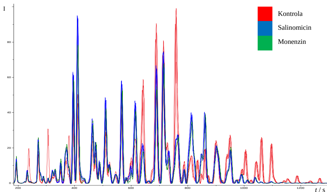
Slika 18. Usporedba kromatograma tripplikata sekretiranih N-glikana HMLE-pBp stanične linije kontrole (crveno) te HMLE-pBp stanične linije nakon tretmana salinomicinom (plavo) i monenzinom (zeleno).
