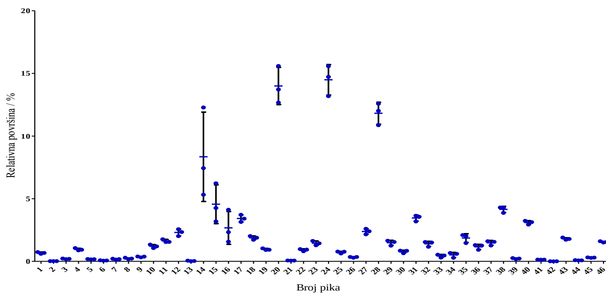
Slika 16. Odnos relativnih površina unutar triplikata kontrolnih uzoraka za HMLE-pBp staničnu liniju.
