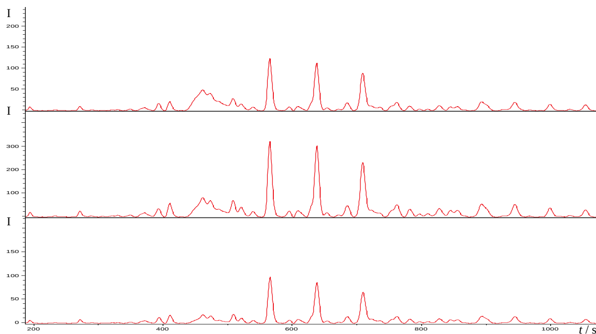
Slika D7. Kromatogrami tehničkih triplikata slobodnih glikana obilježenih prokainamidom iz sekretoma kontrole HMLE-Twist stanične linije uz fluorescentnu detekciju pri 370 nm
