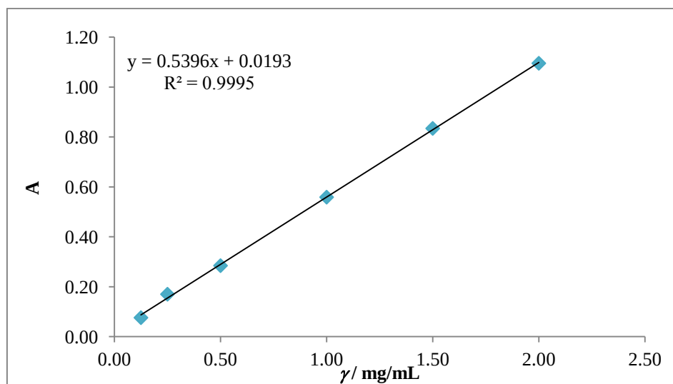
Slika D3. Baždarni dijagram dobiven mjerenjem poznatih masenih koncentracija albumina iz goveđeg seruma (BSA) prema tablici 4. te pripadajuća jednačba pravca prema kojoj je određena nepoznata koncentracija proteina u sekretumu stanične linije HMLE-Twist.
