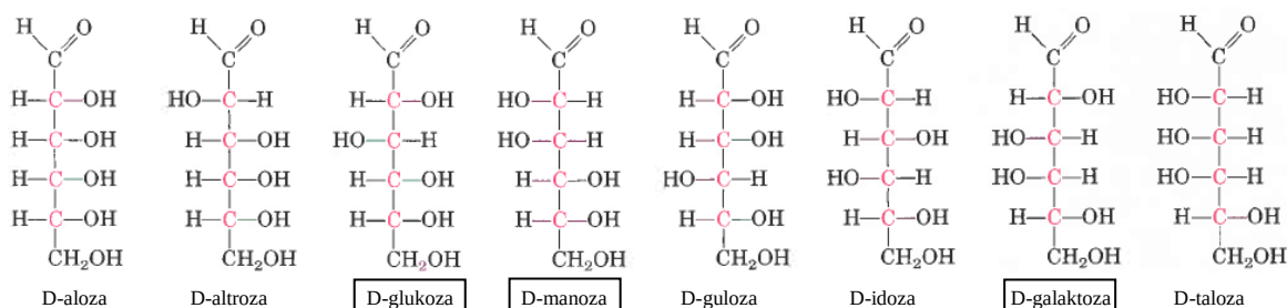
Slika 5. Niz D-aldoza sa šest C atoma. Imena u kvadratićima se najčešće pojavljuju u biološkim sustavima. Kiralni C atomi su označeni crvenom bojom. (preuzeto i modificirano iz ref. 21)
