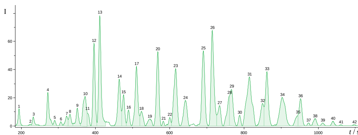
Slika D10. Kromatogram slobodnih glikana obilježenih prokainamidom iz sekretoma nakon tretmana monenzinom HMLE-pBp stanične linije. Fluorescentna detekcija pri valnoj duljini od 370 nm
