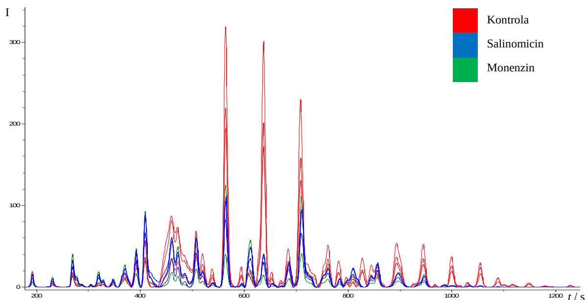
Slika 19. Usporedba kromatograma tripplikata sekretiranih N-glikana HMLE-Twist stanične linije kontrole (crveno) te HMLE-Twist stanične linije nakon tretmana salinomicinom (plavo) i duplikata tretiranih monenzinom (zeleno).
