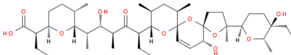
Slika 2. Struktura salinomicina (SAL). (preuzeto iz ref. 22)
