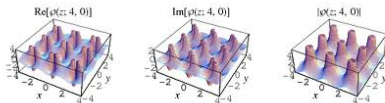
Slika 2.2: Grafovi funkcije \varphi(z)
