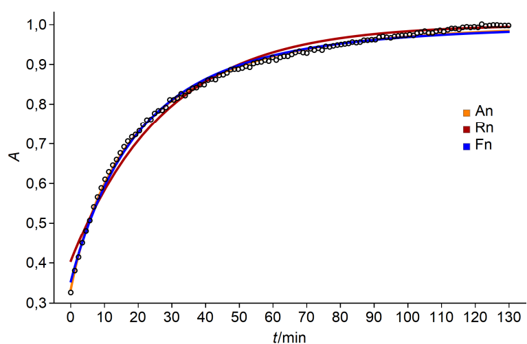
Slika 40. Teorijske kinetičke krivulje dobivene nelinearnom regresijskom analizom prema modelima An, Fn i Rn za reakciju nastajanja azodioksida spoja 1 pri 230 K.
