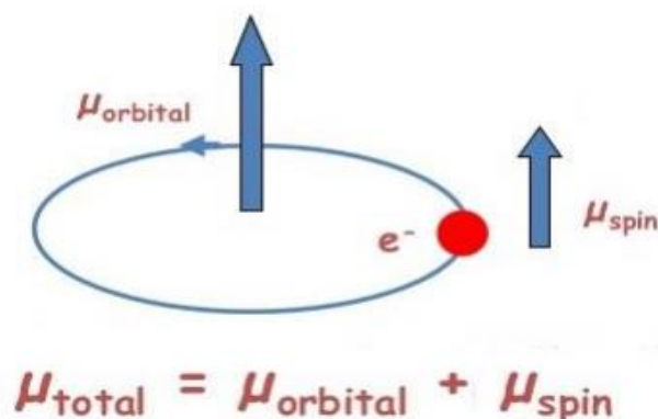
Slika 16. Smjer i doprinos spinskog ( \mu_s ) i orbitalnog ( \mu_L ) magnetskog momenta
