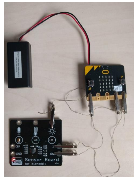
Slika 19. Poslije spajanja
