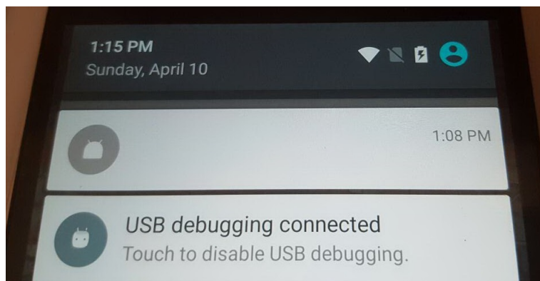
Slika 7.5: Prazna obavijest
