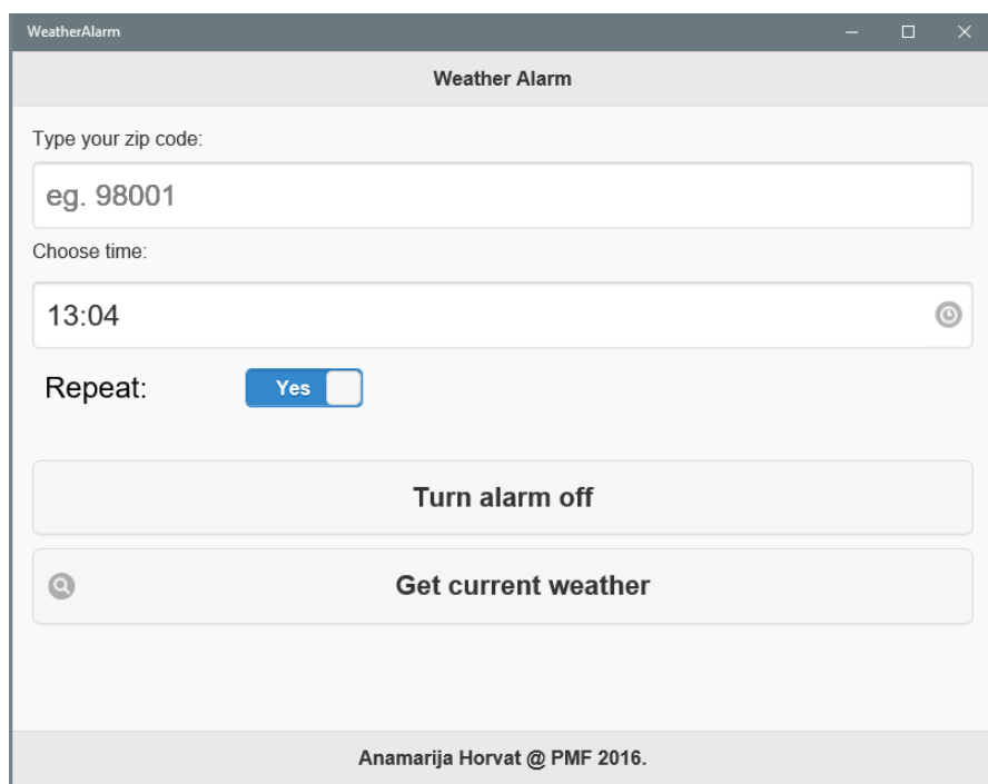
Slika 8.3: Windows aplikacije
